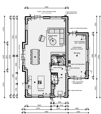
Begane grond v.z.v. vloerverwarming exclusief berging
