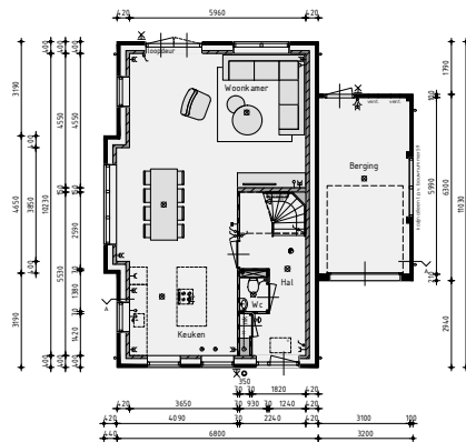
Begane grond v.z.v. vloerverwarming exclusief berging
