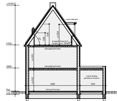
Principe doorsnede A-A
