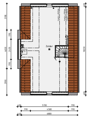
2de Verdieping v.z.v. vloerverwarming
