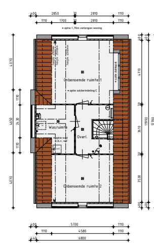
2de Verdieping v.z.v. vloerverwarming
