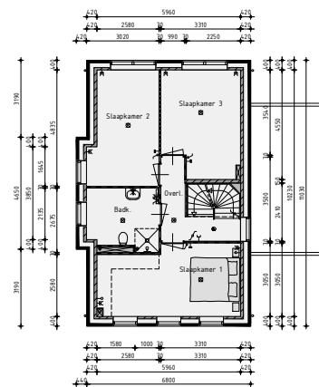
1ste Verdieping v.z.v. vloerverwarming
