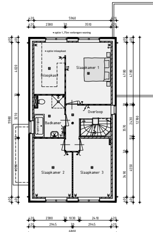
1ste Verdieping v.z.v. vloerverwarming
