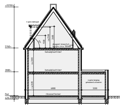
Principe doorsnede A-A
