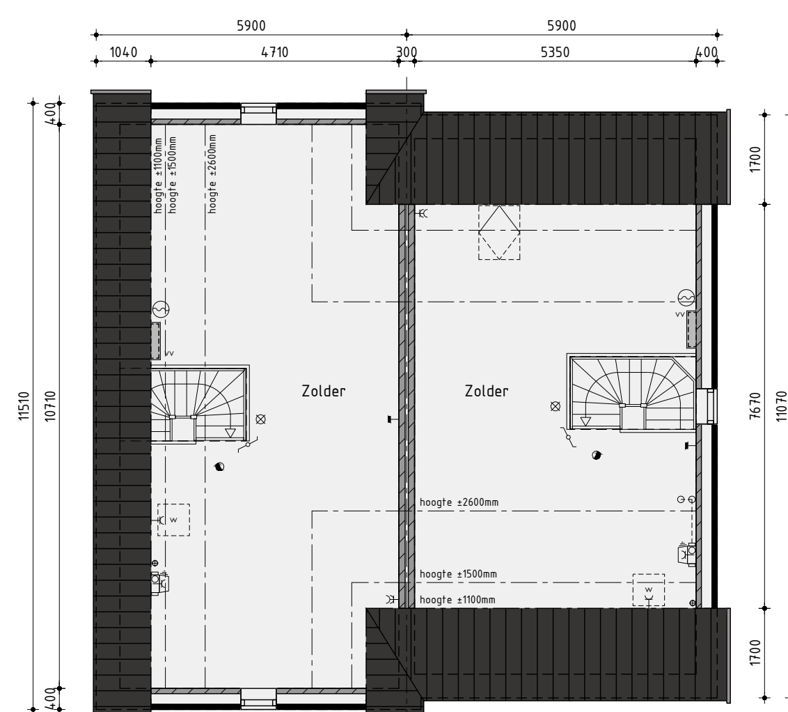
2de Verdieping
