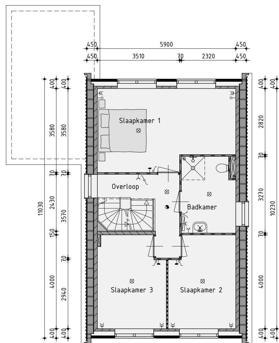
1ste Verdieping
