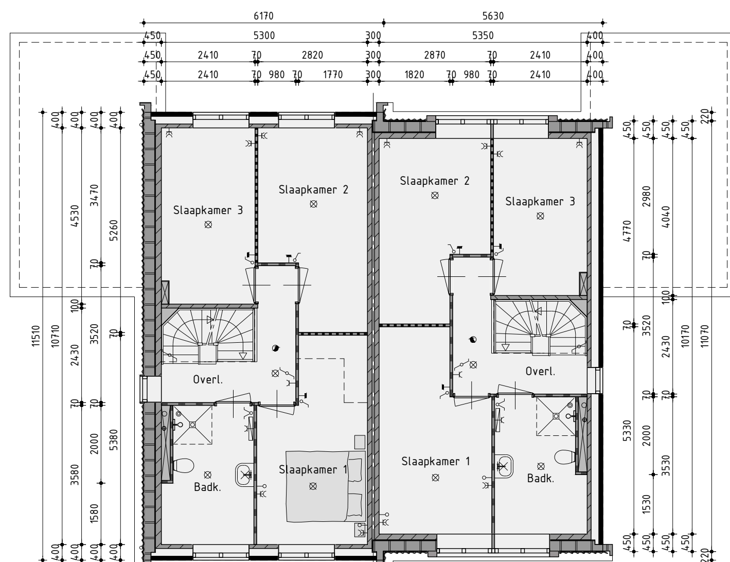
1ste Verdieping
