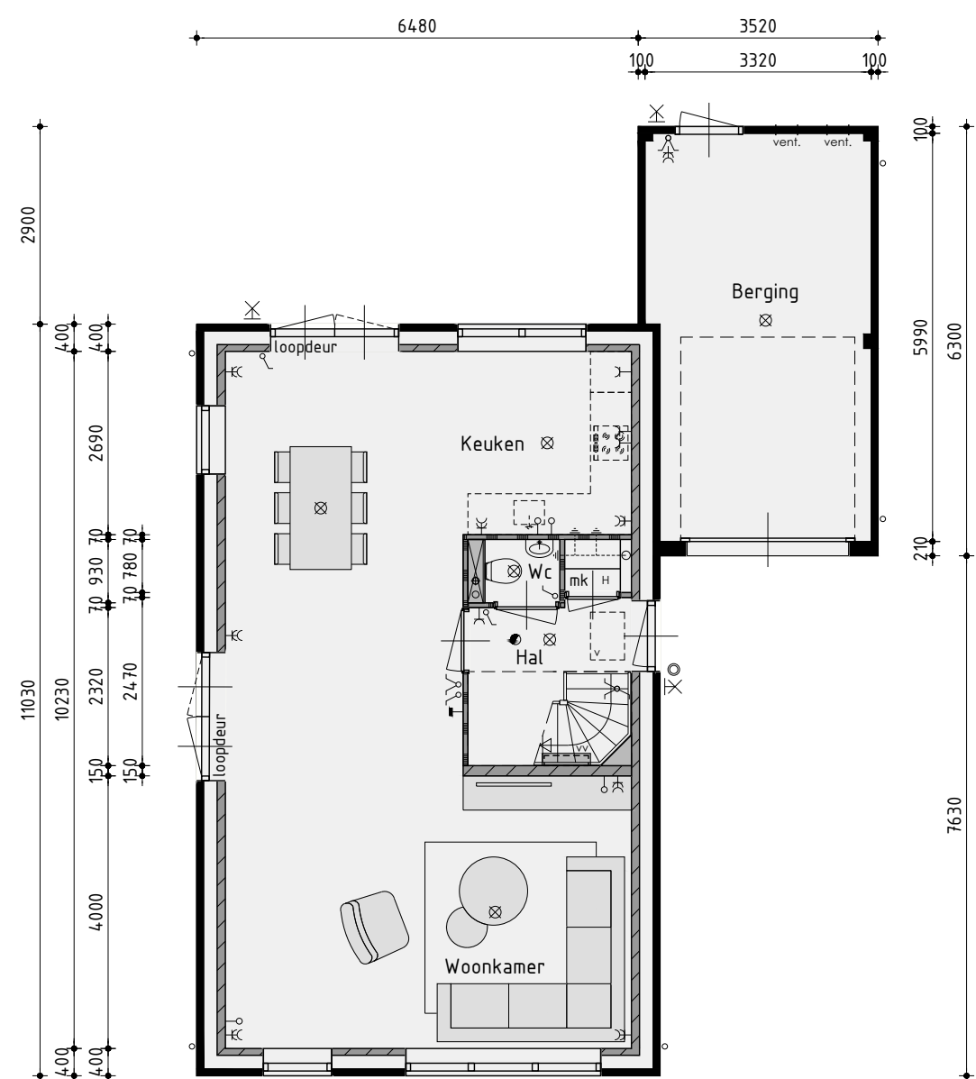
Begane grond
