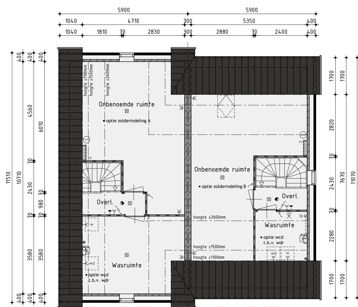
2de Verdieping v.z.v. vloerverwarming
