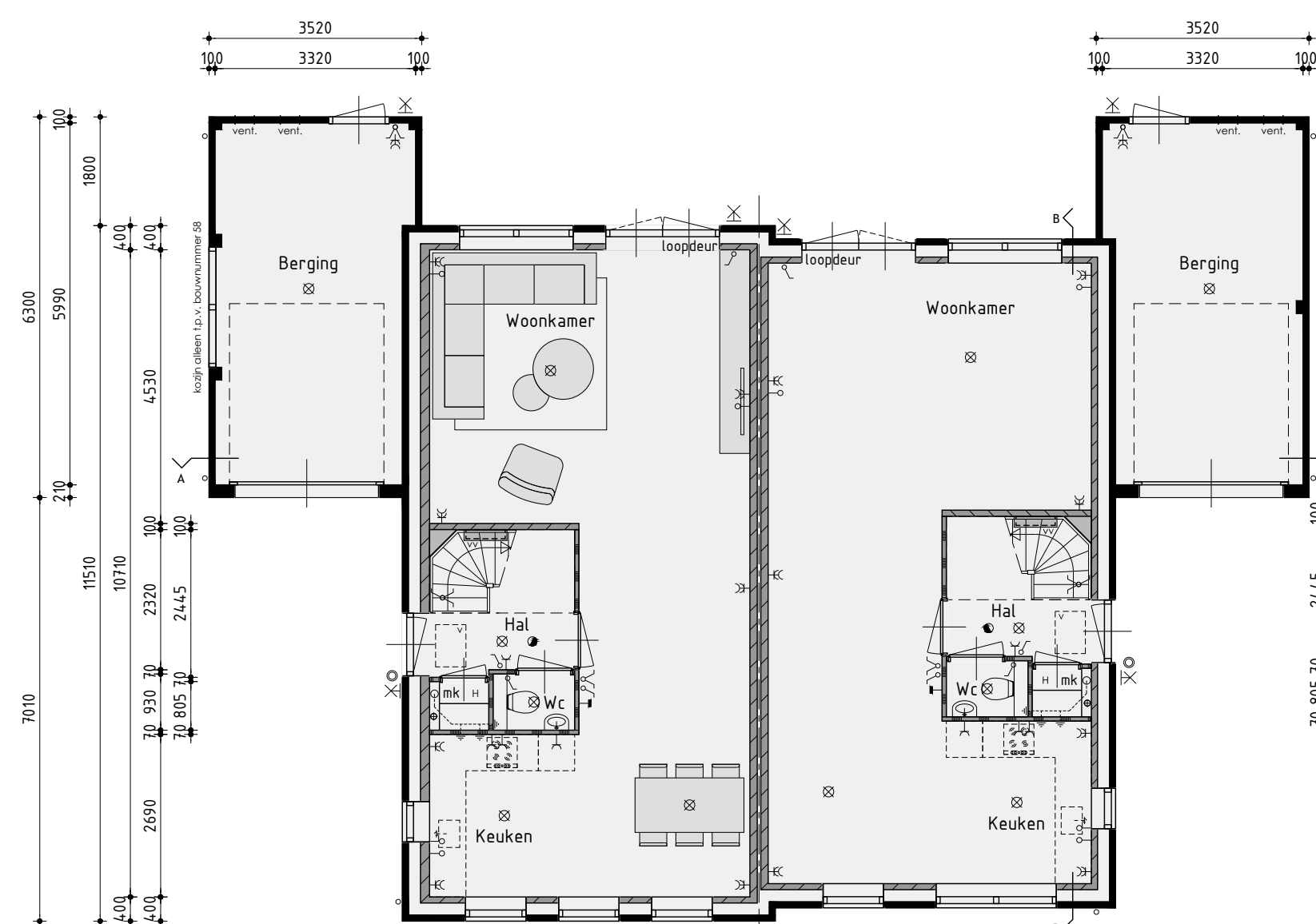
Begane grond
