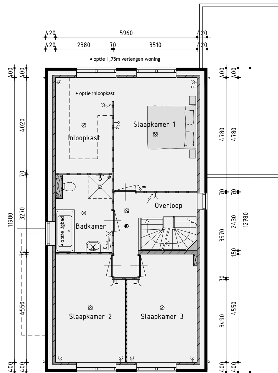
1ste Verdieping
