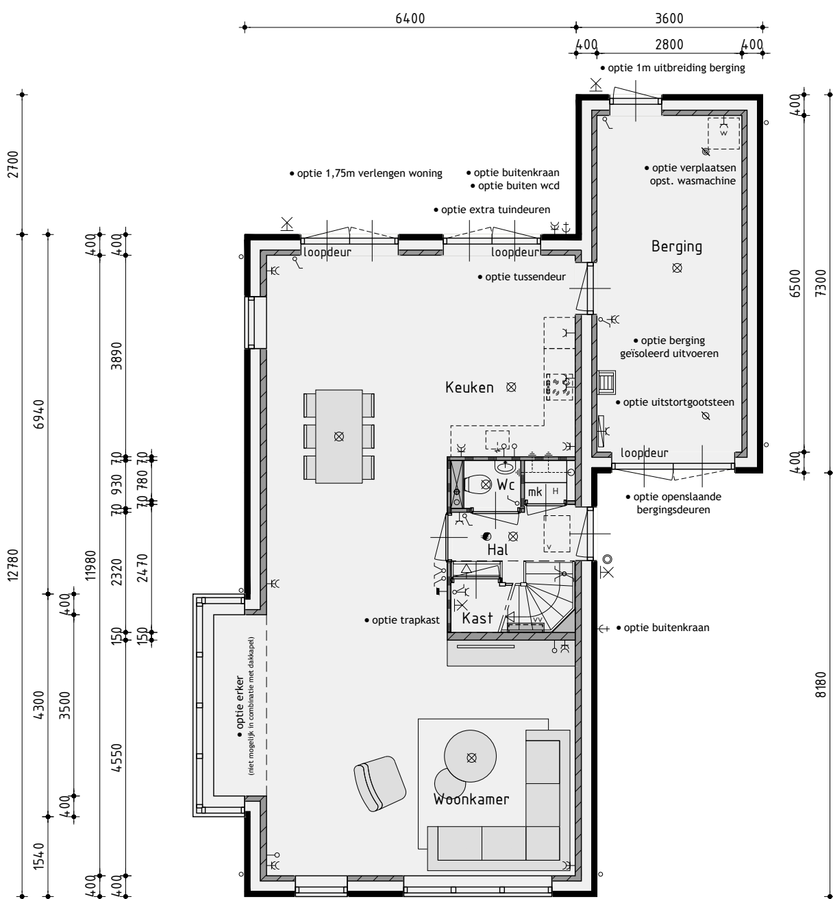
Begane grond
