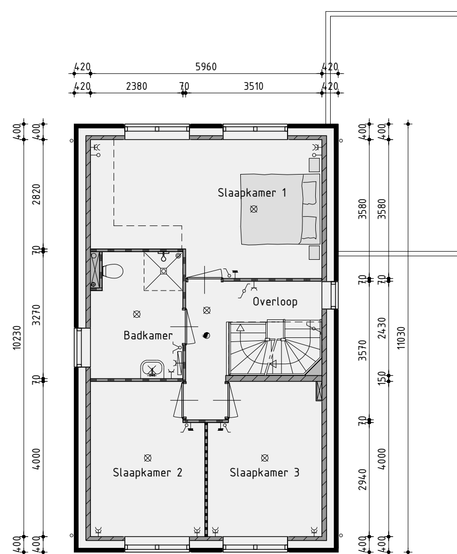
1ste Verdieping
