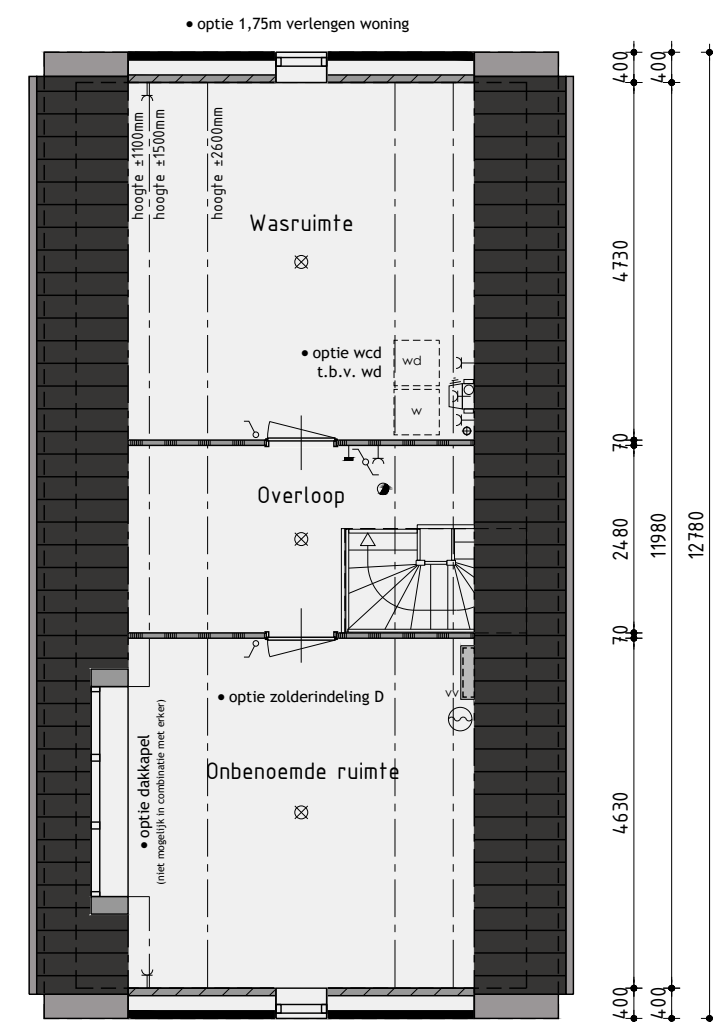
2de Verdieping
