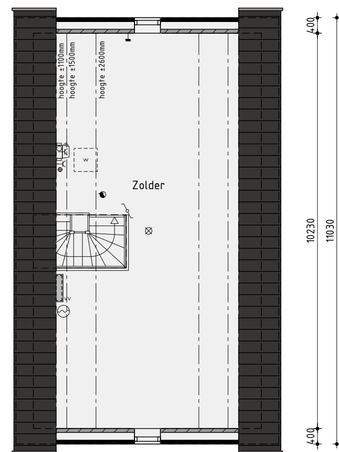
2de Verdieping
