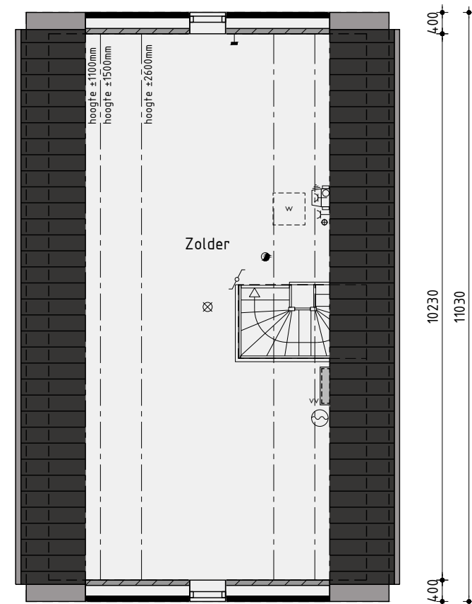
2de Verdieping
