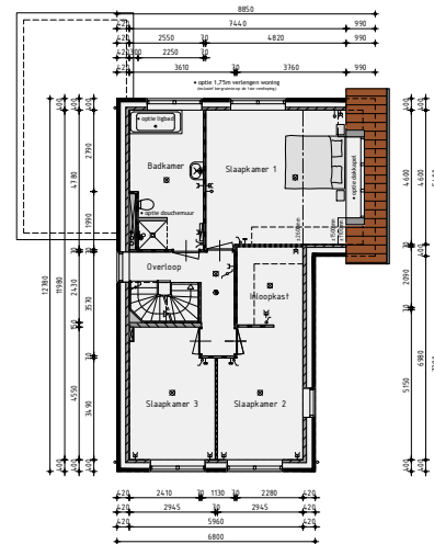
1ste Verdieping v.z.v. vloerverwarming
