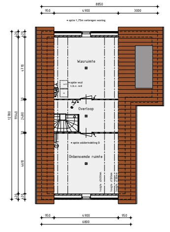
2de Verdieping v.z.v. vloerverwarming
