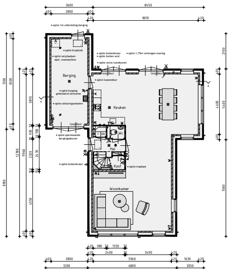
Begane grond v.z.v. vloerverwarming exclusief berging
