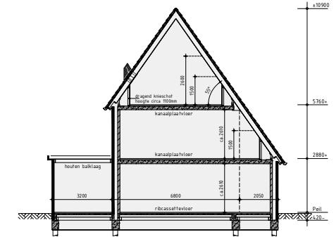
Principe doorsnede B-B
