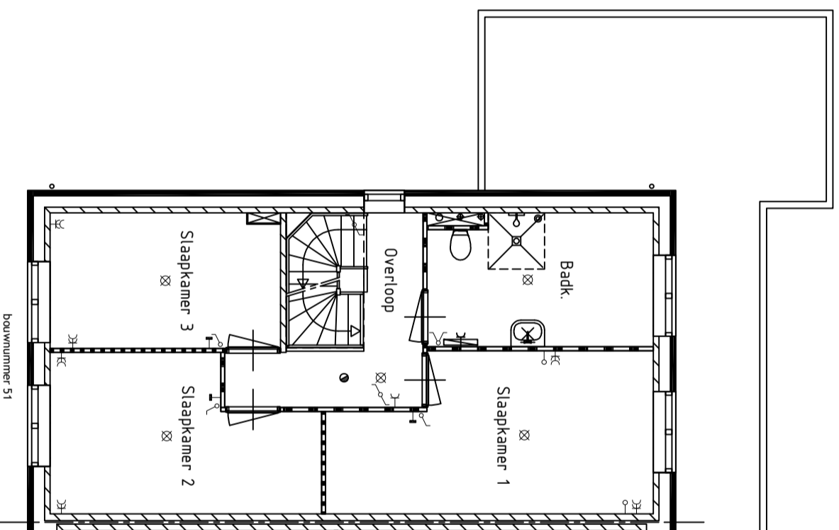
1ste Verdieping
