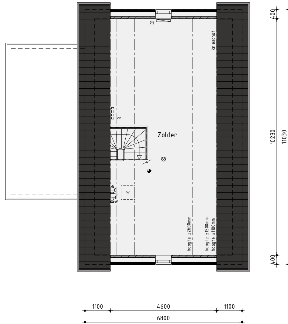
2de Verdieping
