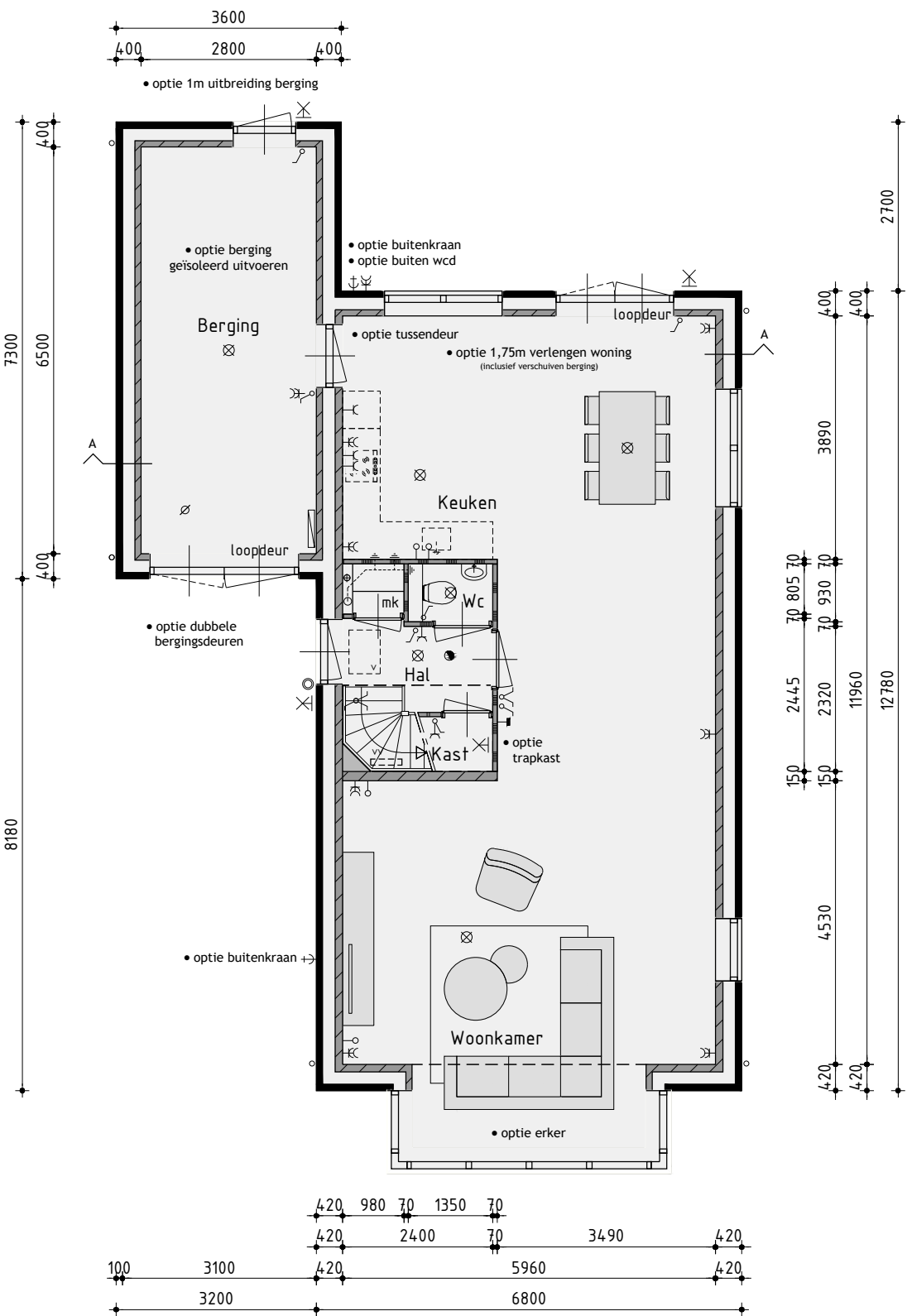
Begane grond
