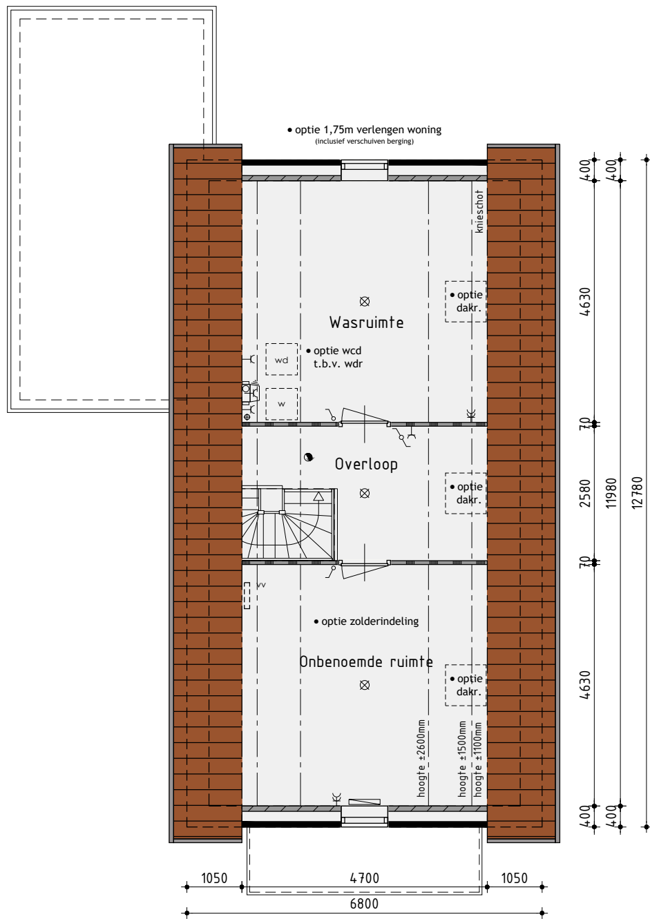
2de Verdieping
