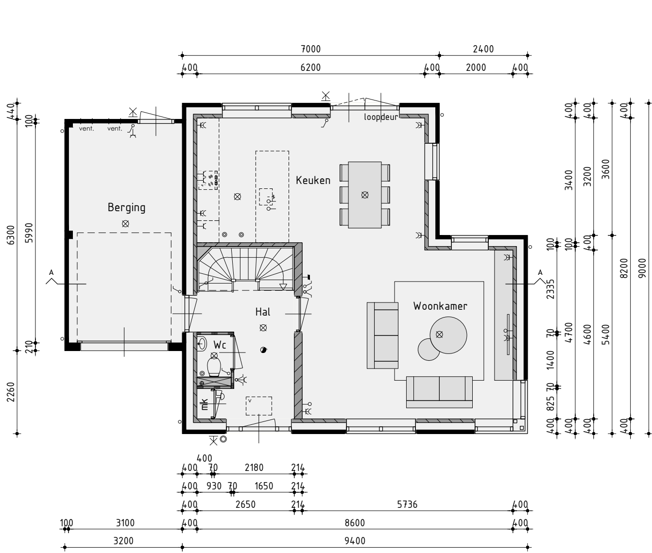
Begane grond
