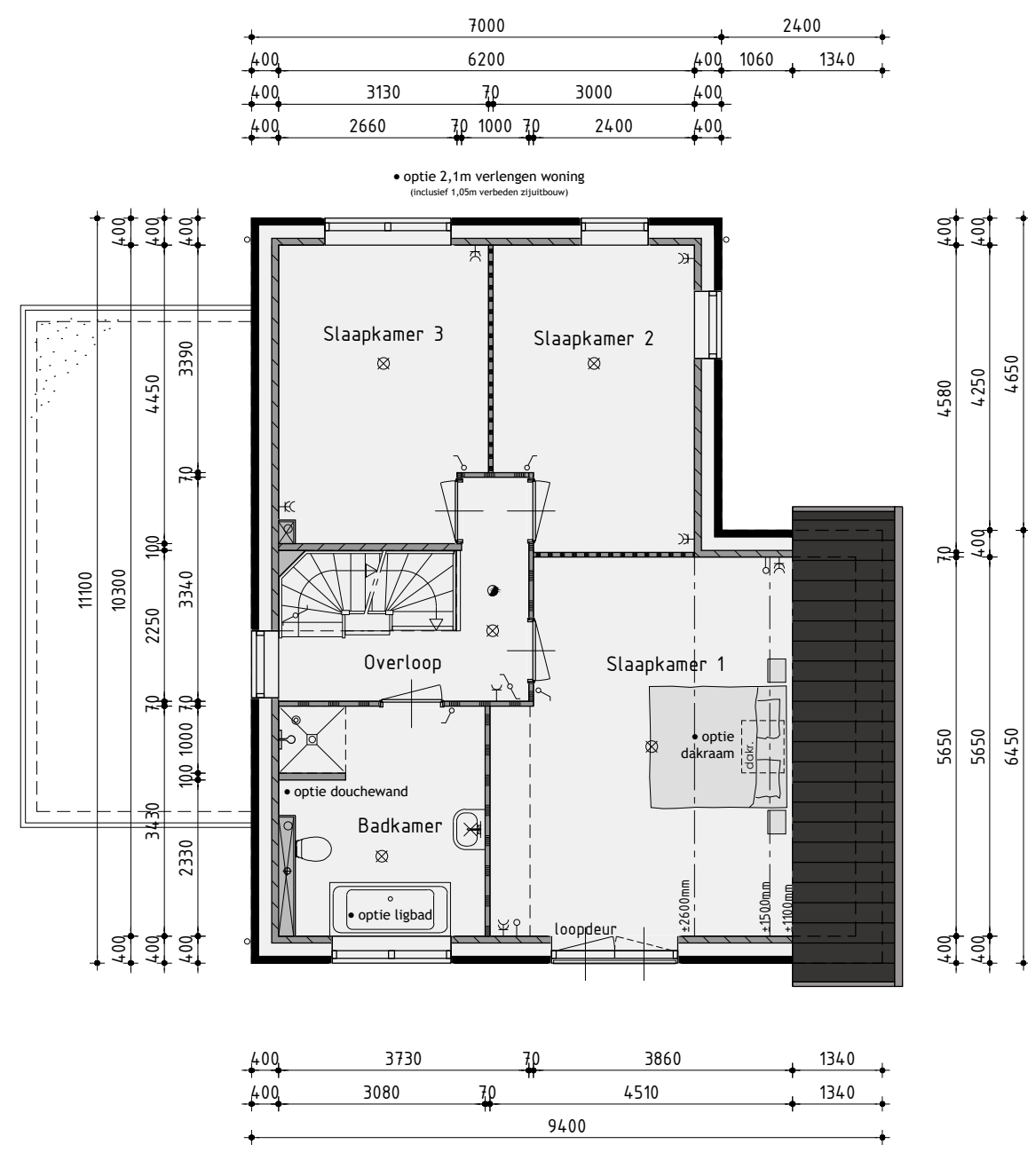
1ste Verdieping
