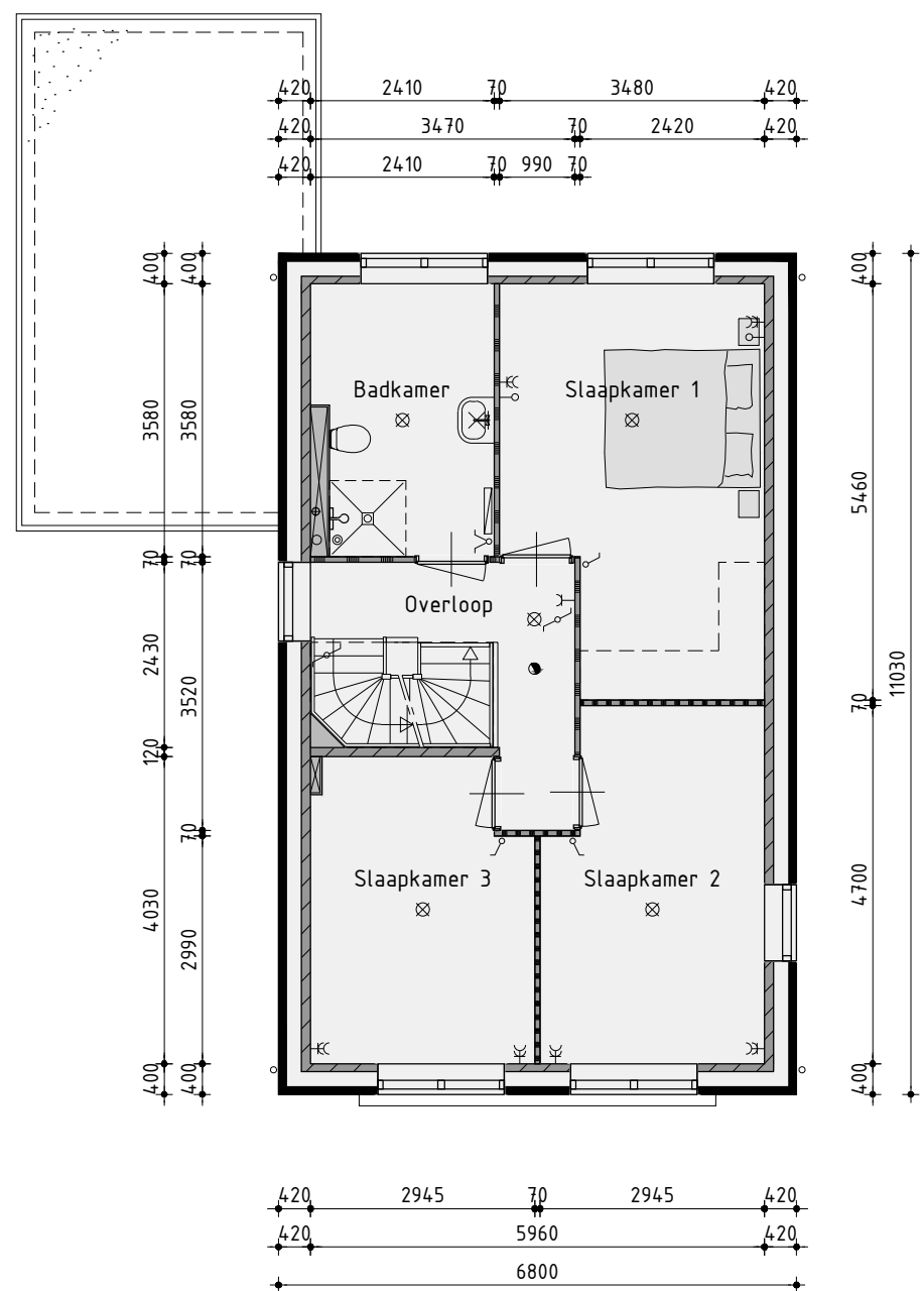
1ste Verdieping
