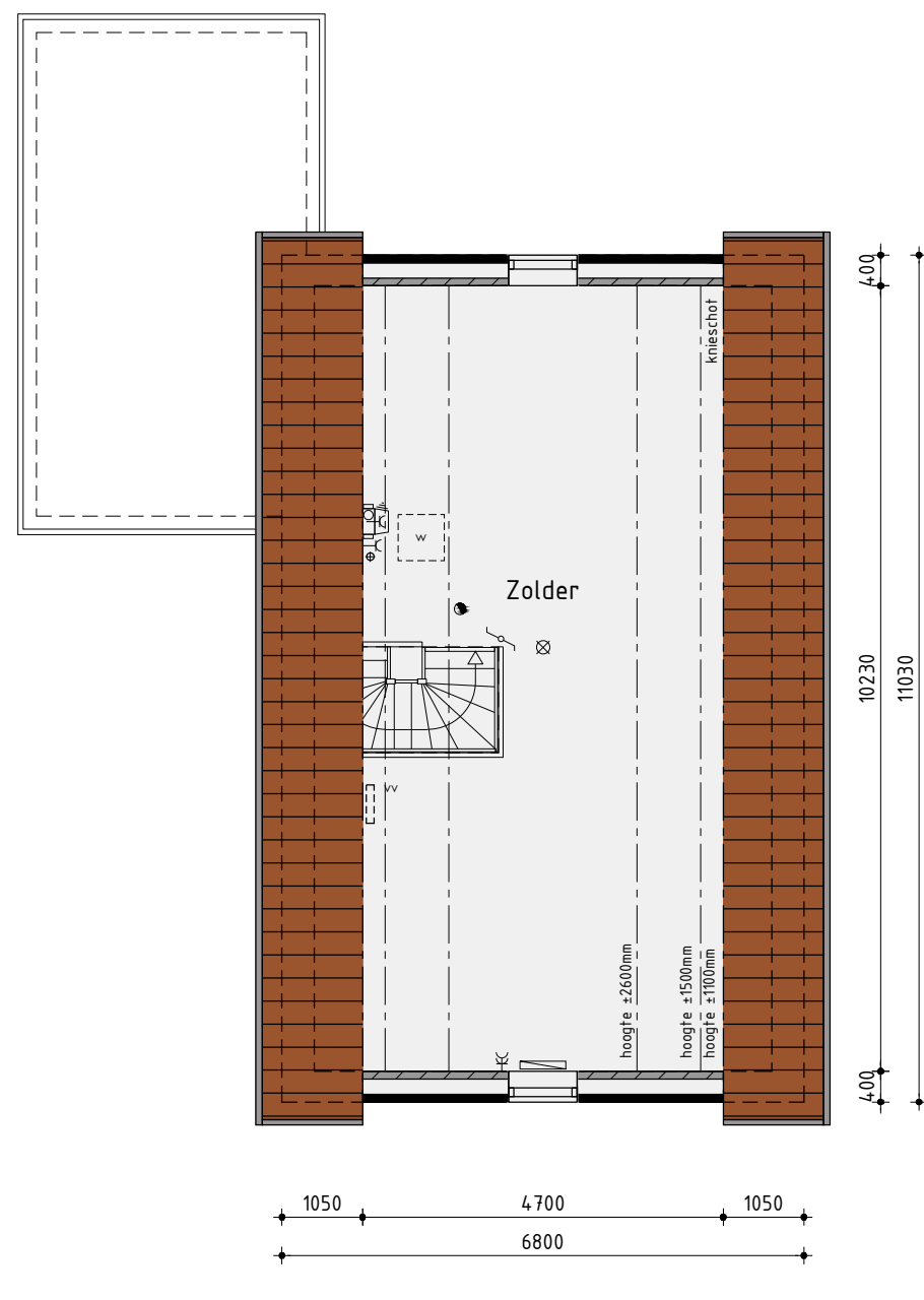
2de Verdieping
