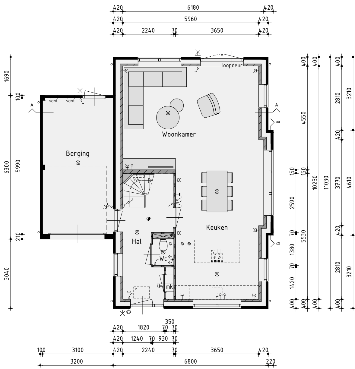
Begane grond
