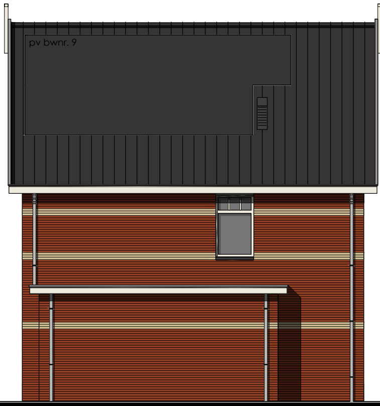
Linker zijgevel
