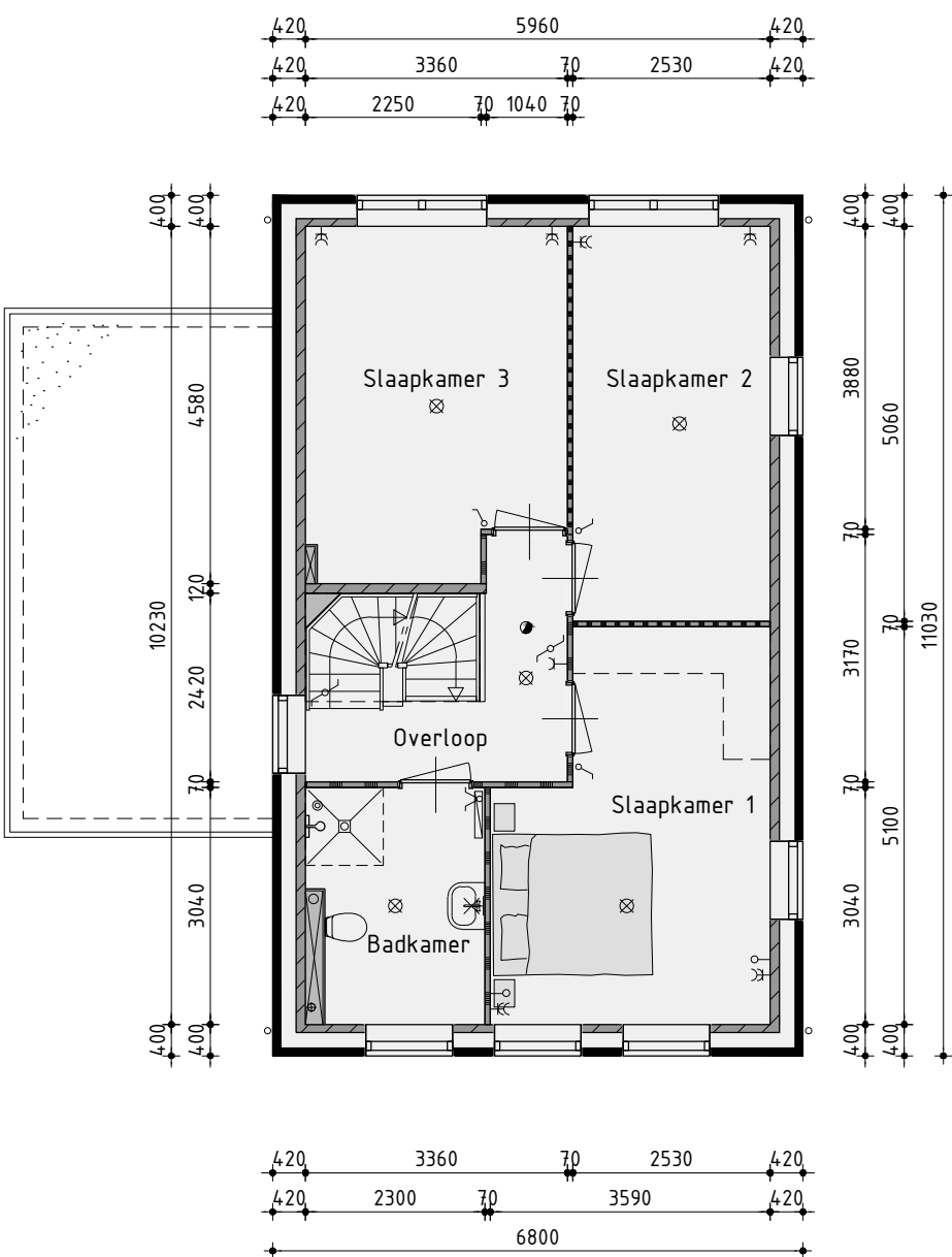
1ste Verdieping
