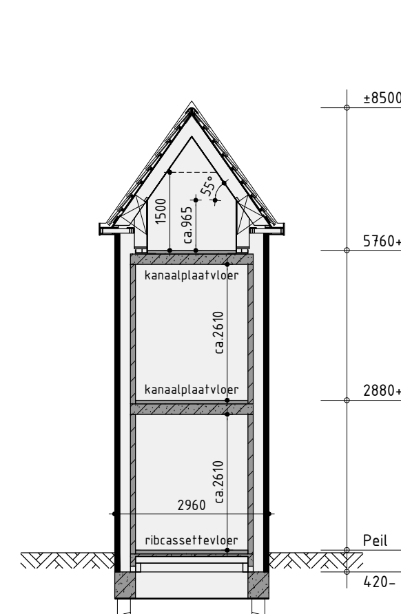
Principe doorsnede D-D
