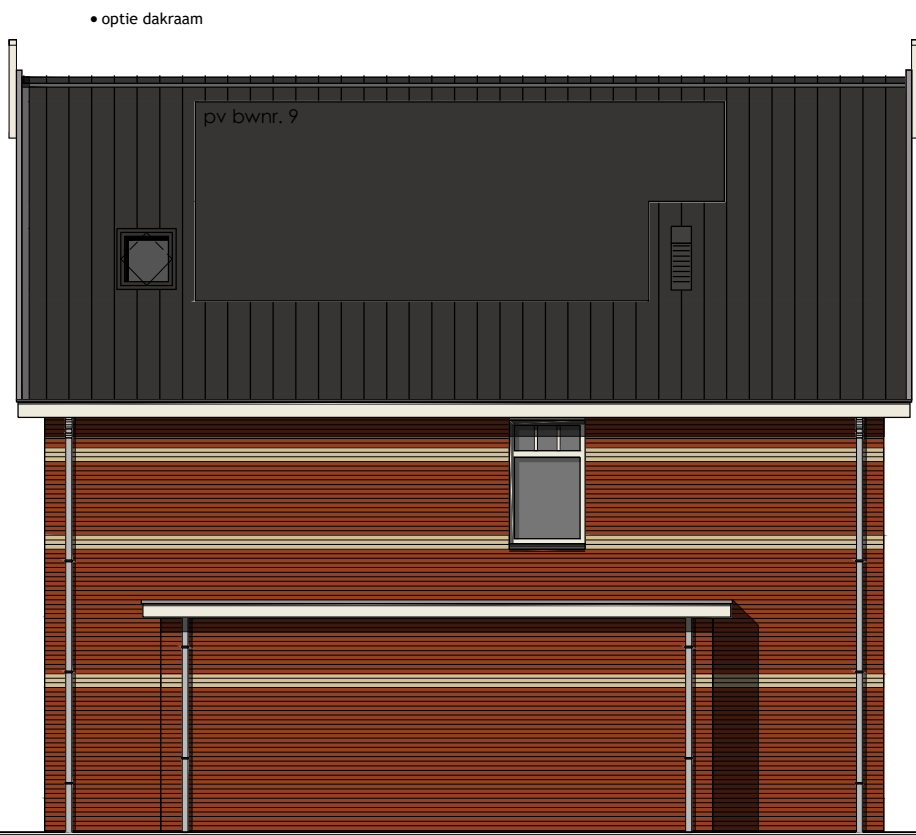
Linker zijgevel
