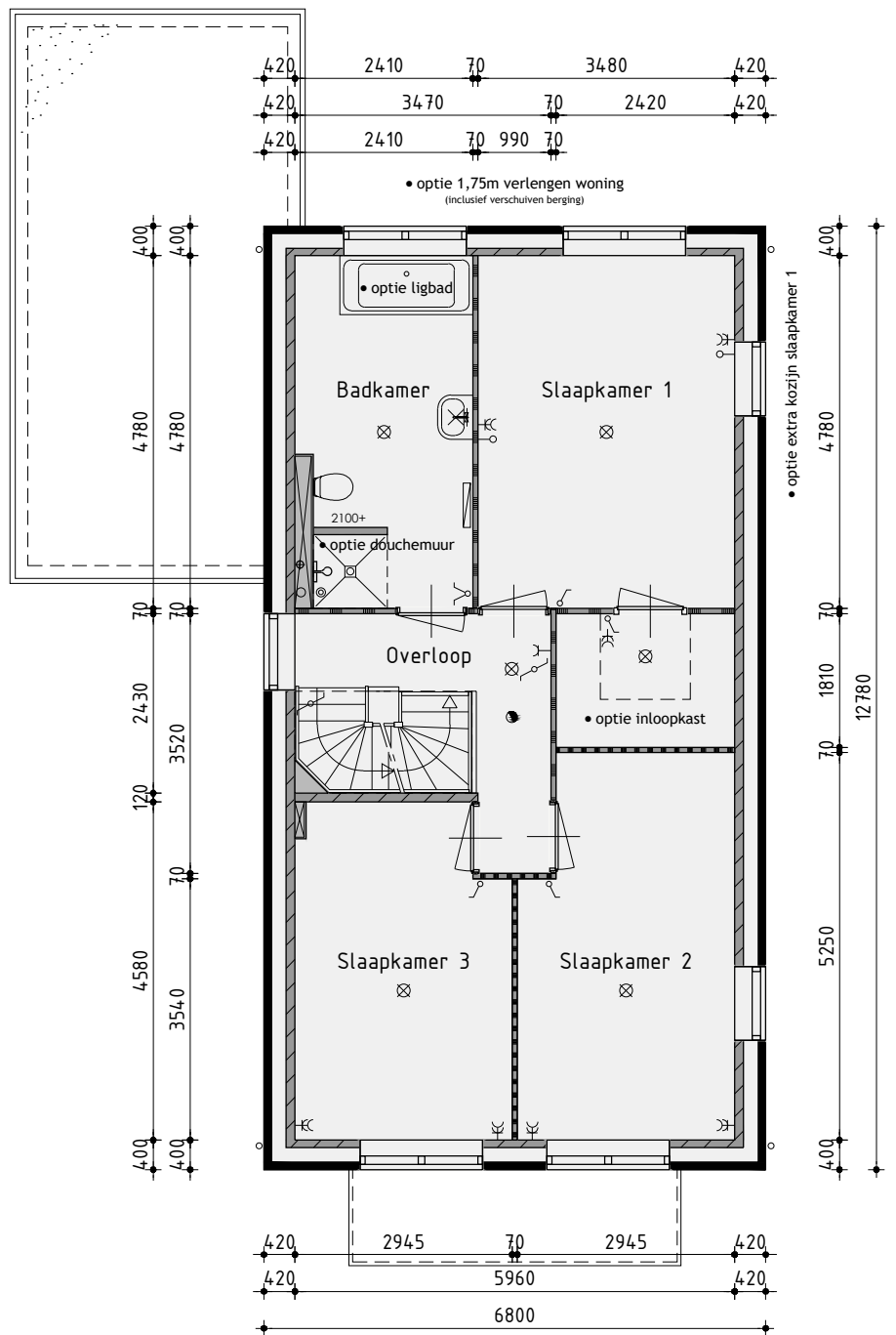
1ste Verdieping
