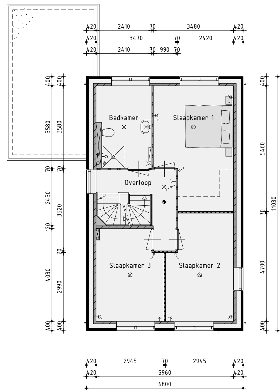
1ste Verdieping
