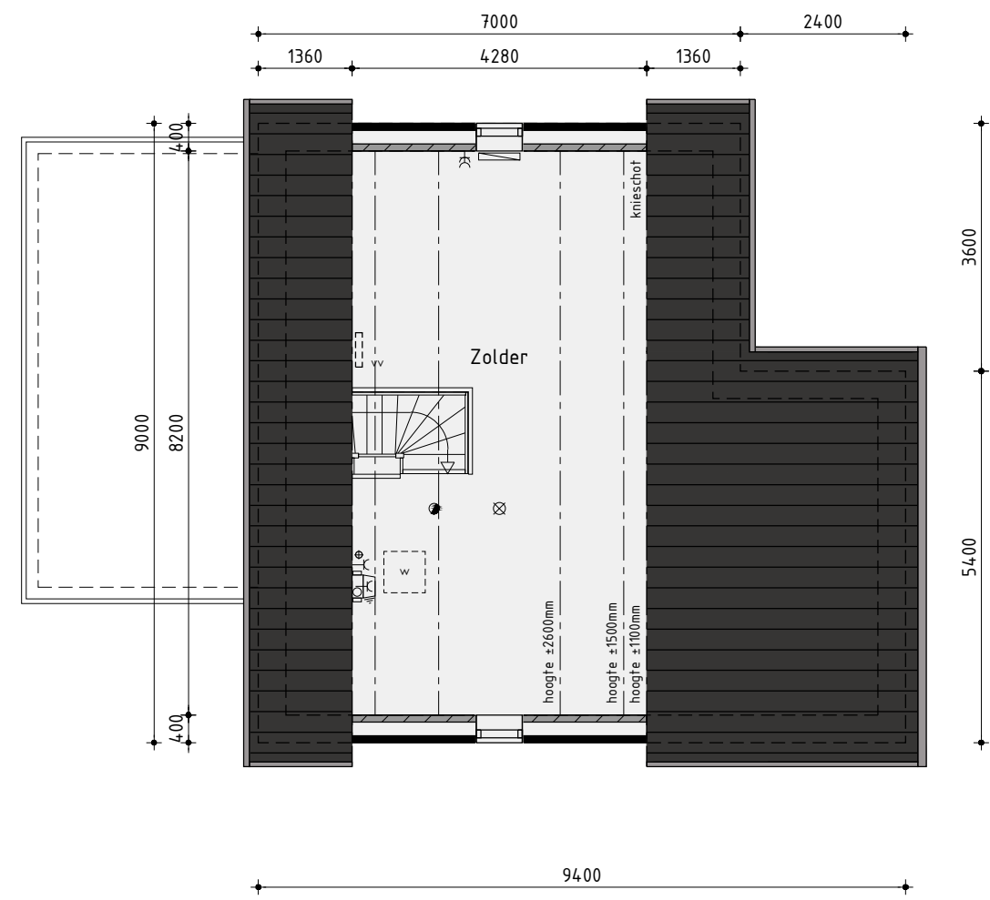
2de Verdieping
