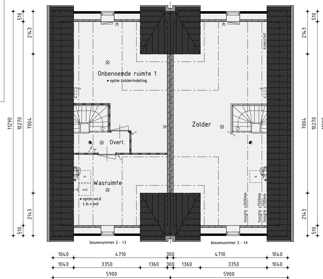
2de Verdieping
