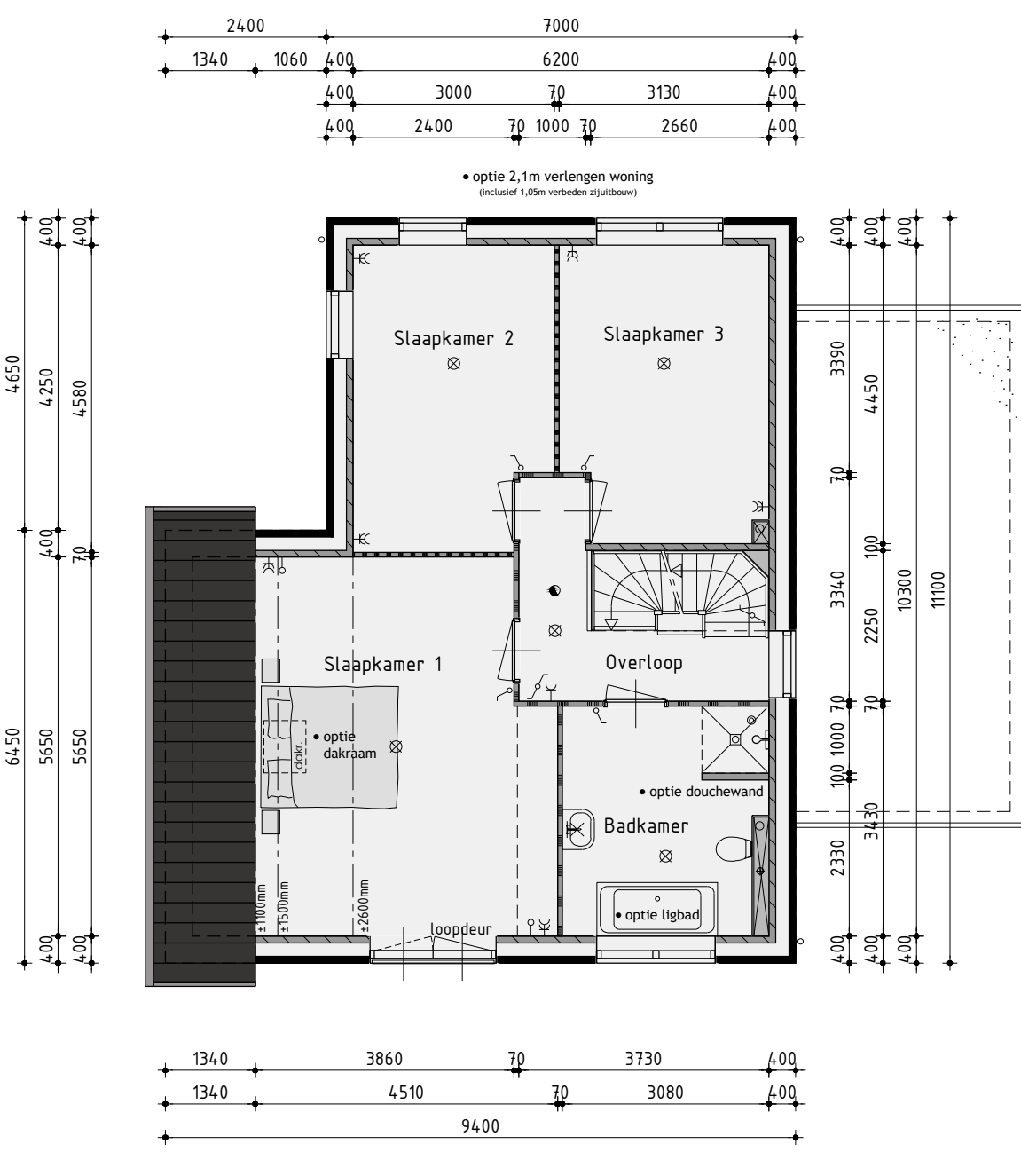
1ste Verdieping
