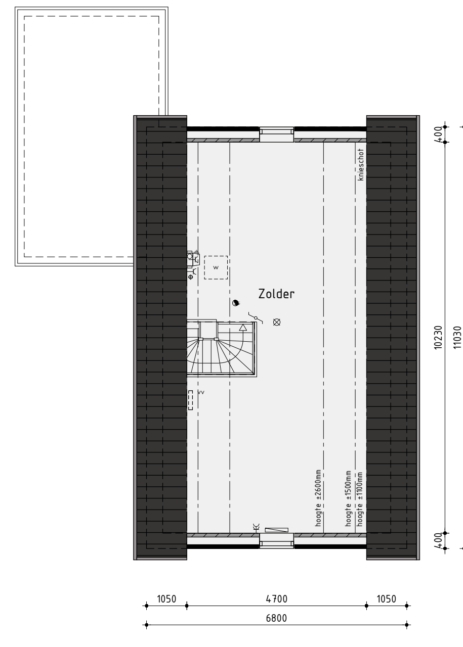
2de Verdieping
