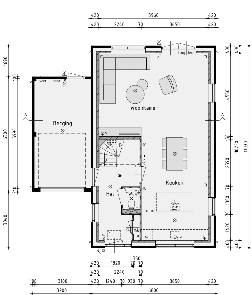
Begane grond
