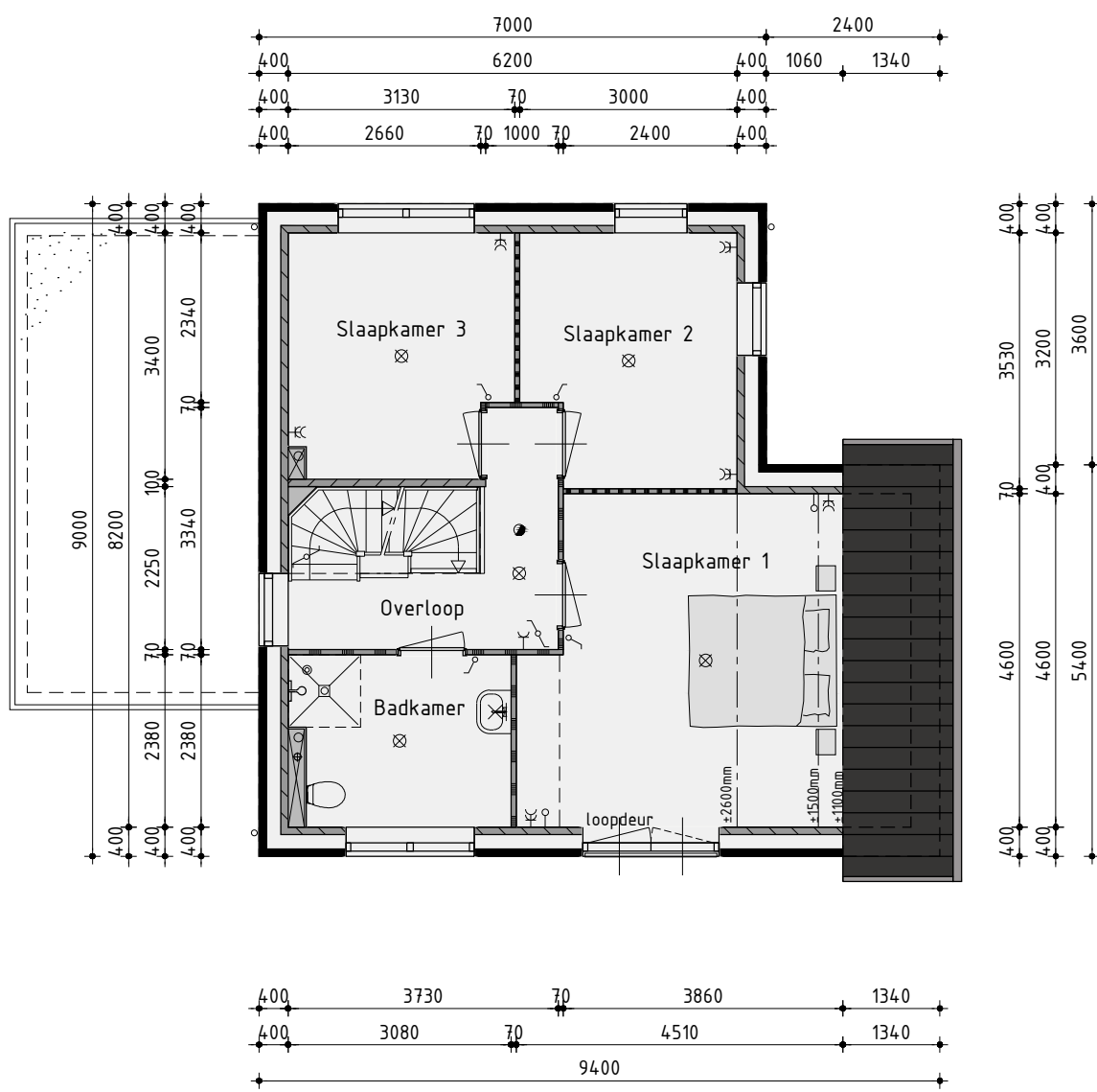
1ste Verdieping
