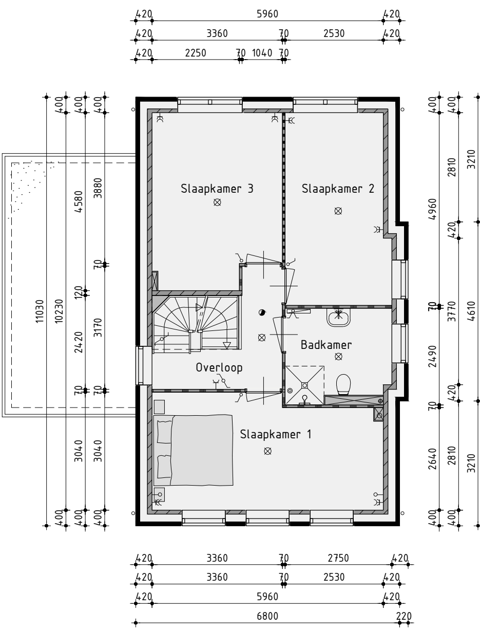
1ste Verdieping
