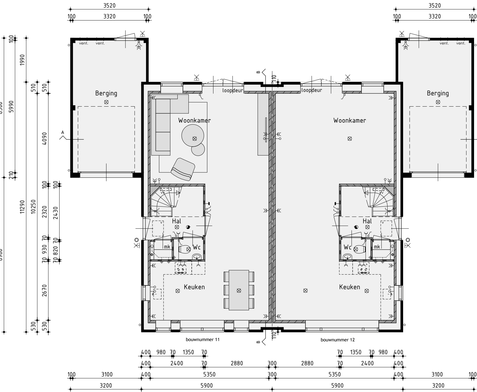
Begane grond
