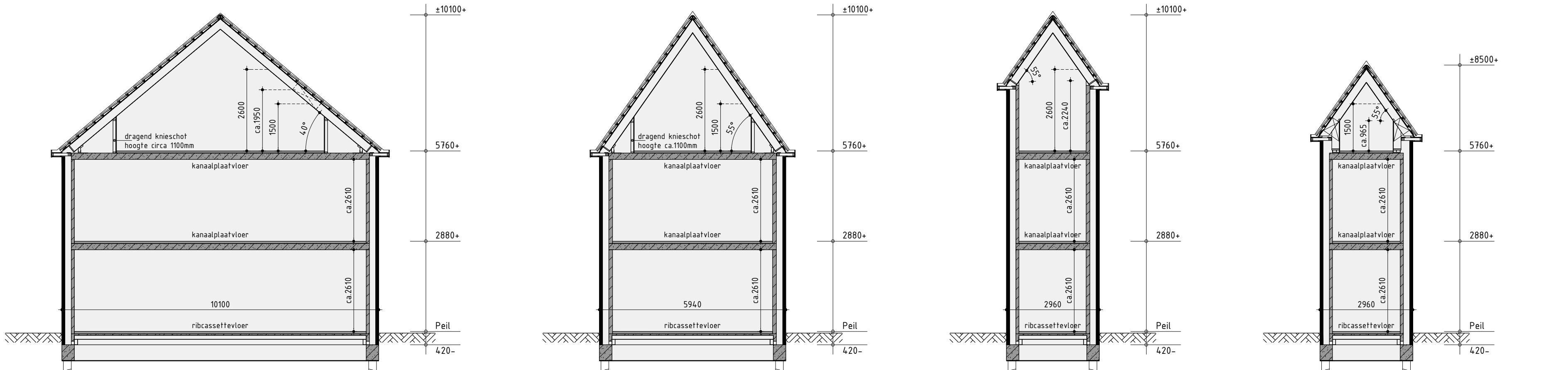
Principe doorsnede A-A
