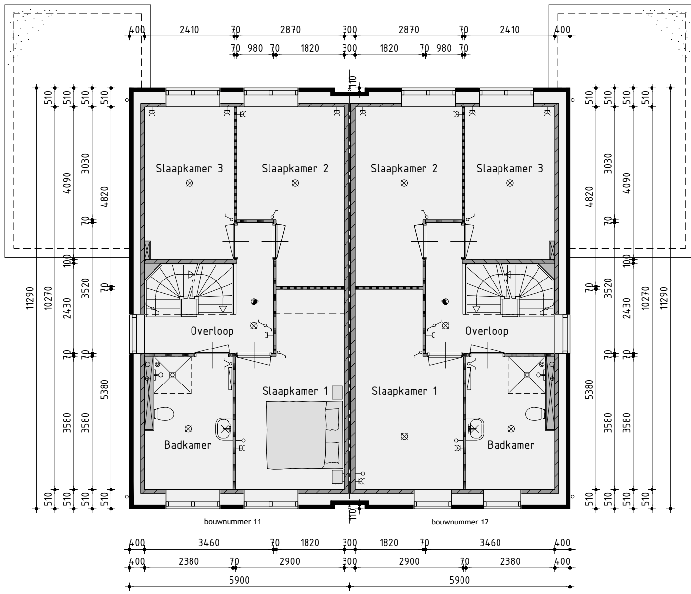
1ste Verdieping
