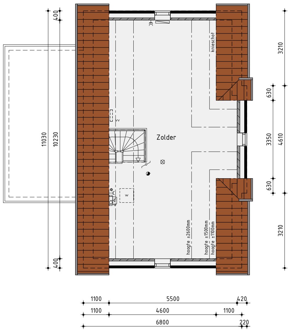
2de Verdieping
