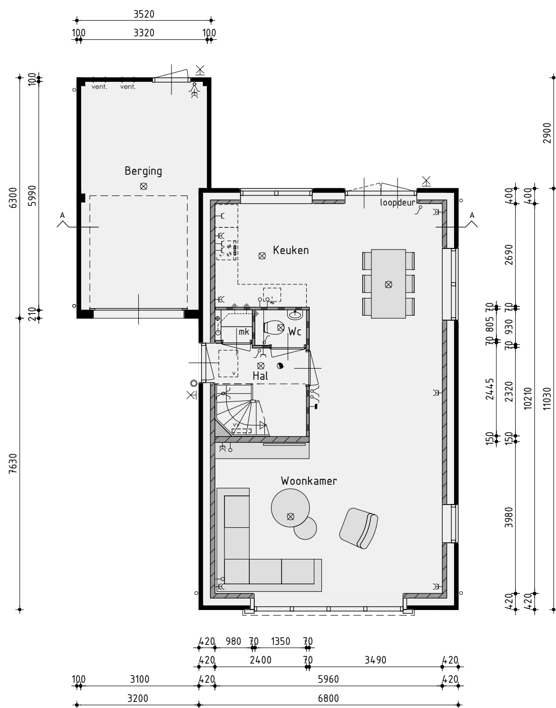
Begane grond
