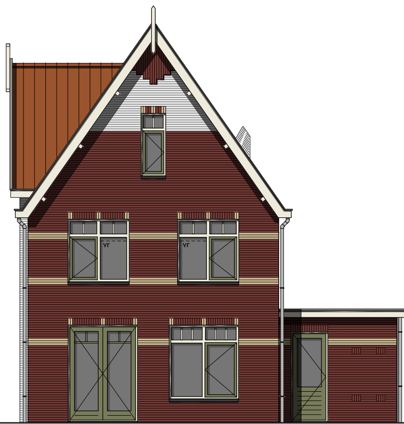
Achtergevel
