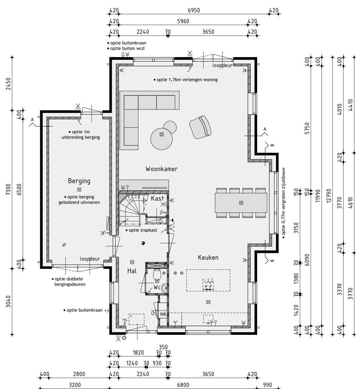
Begane grond
