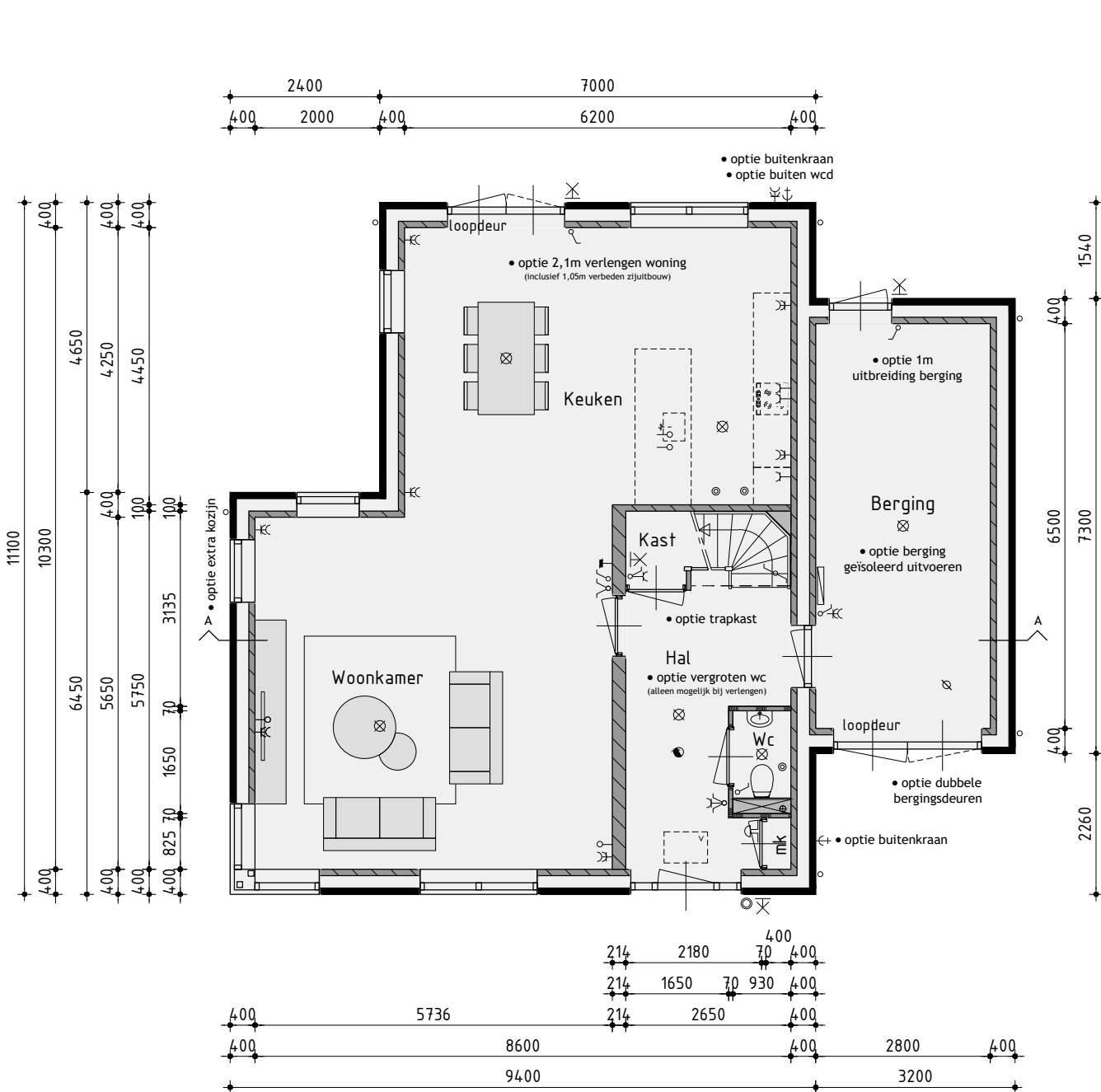
Begane grond
