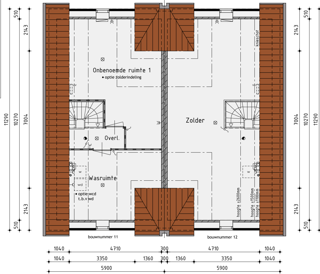
2de Verdieping
