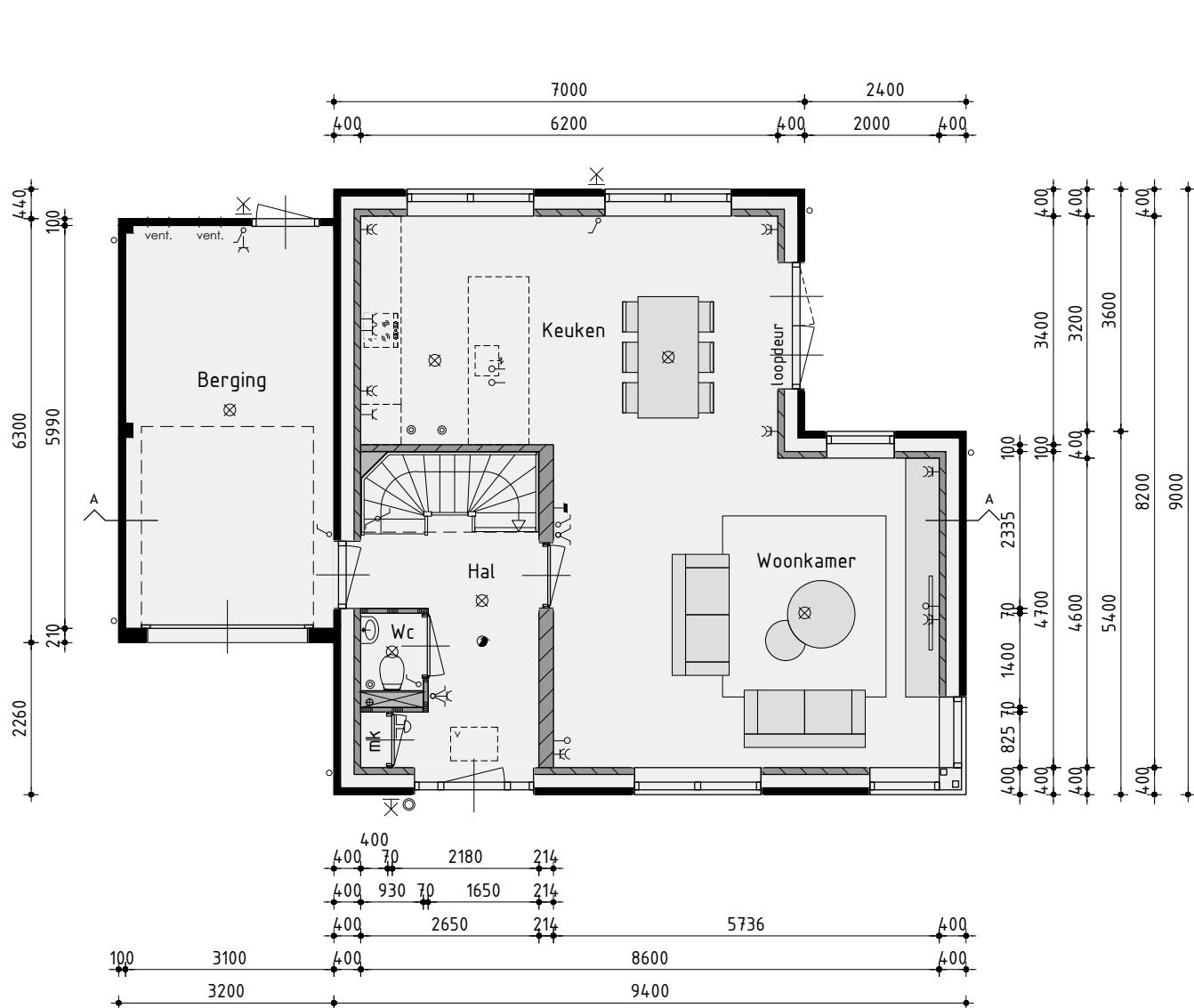
Begane grond
