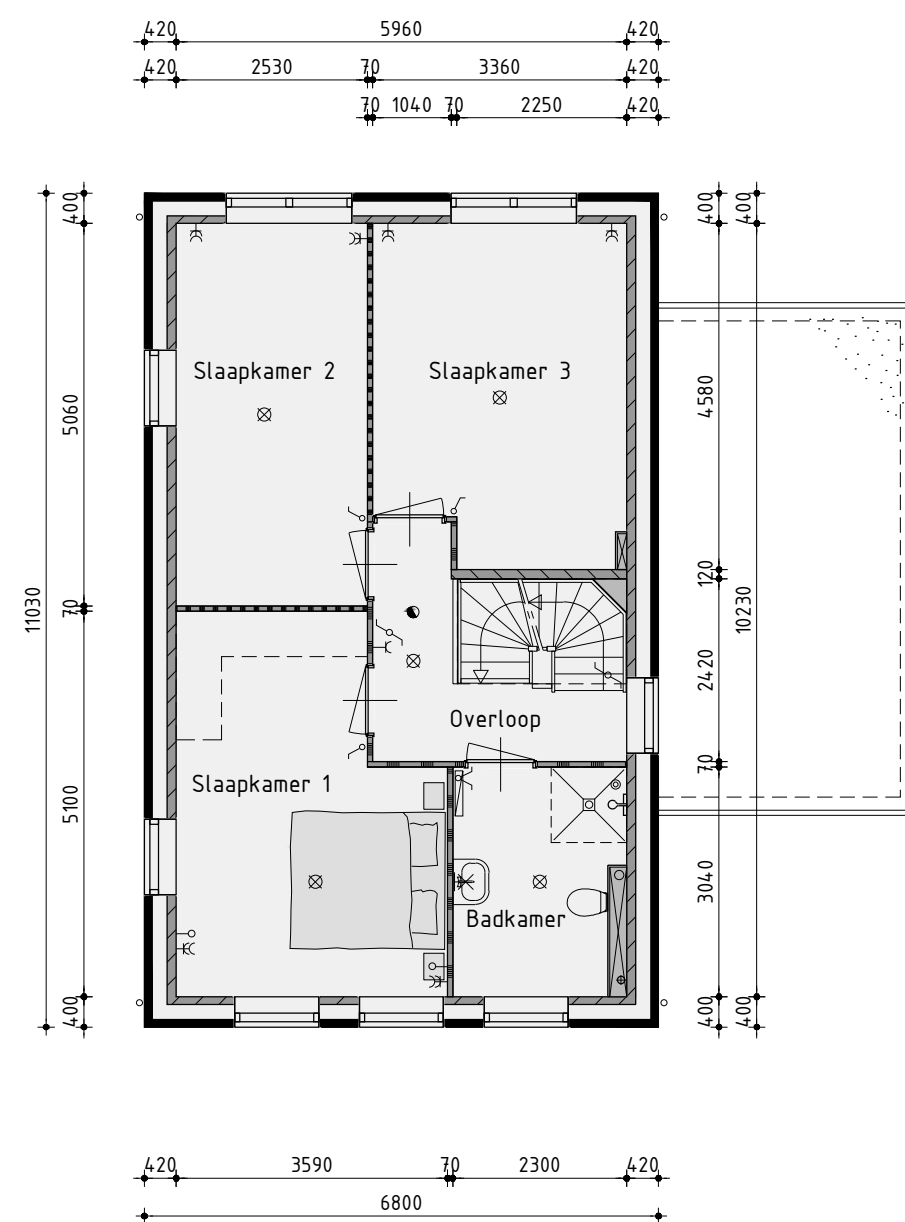
1ste Verdieping
