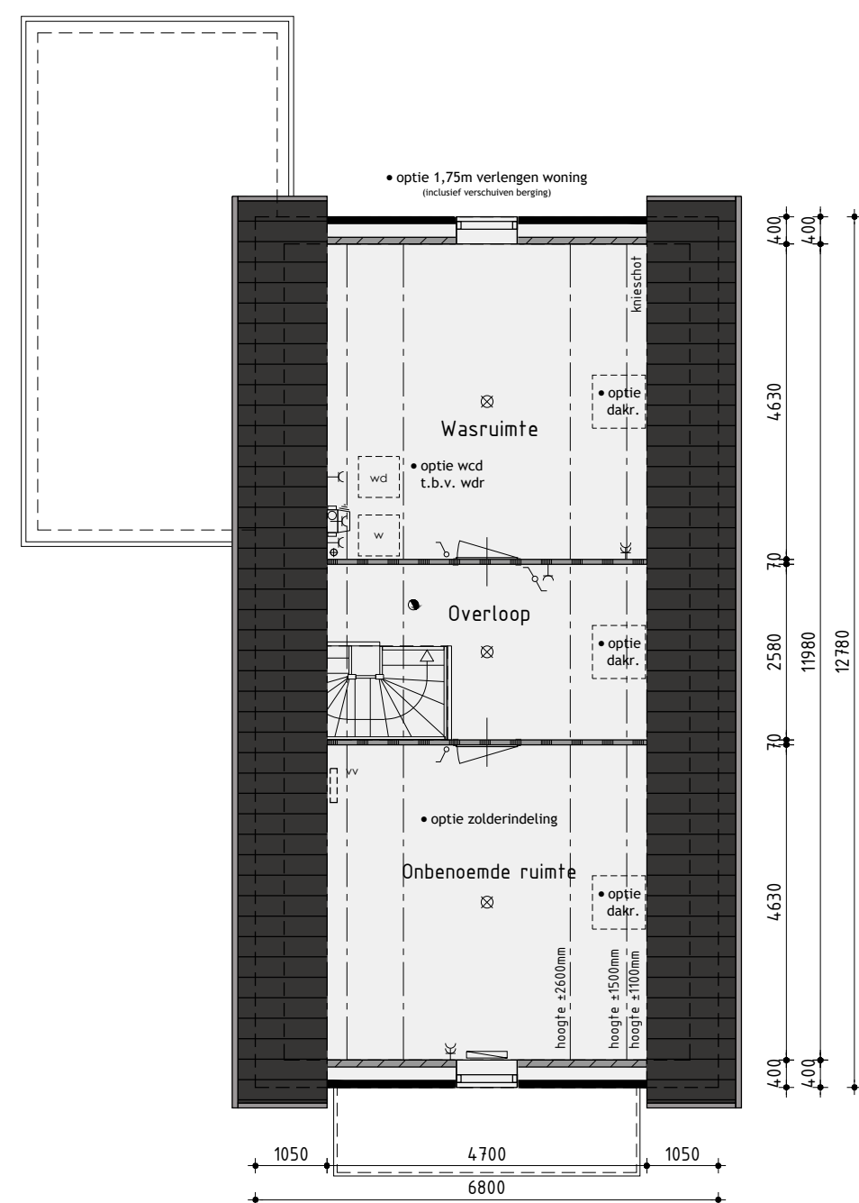
2de Verdieping
