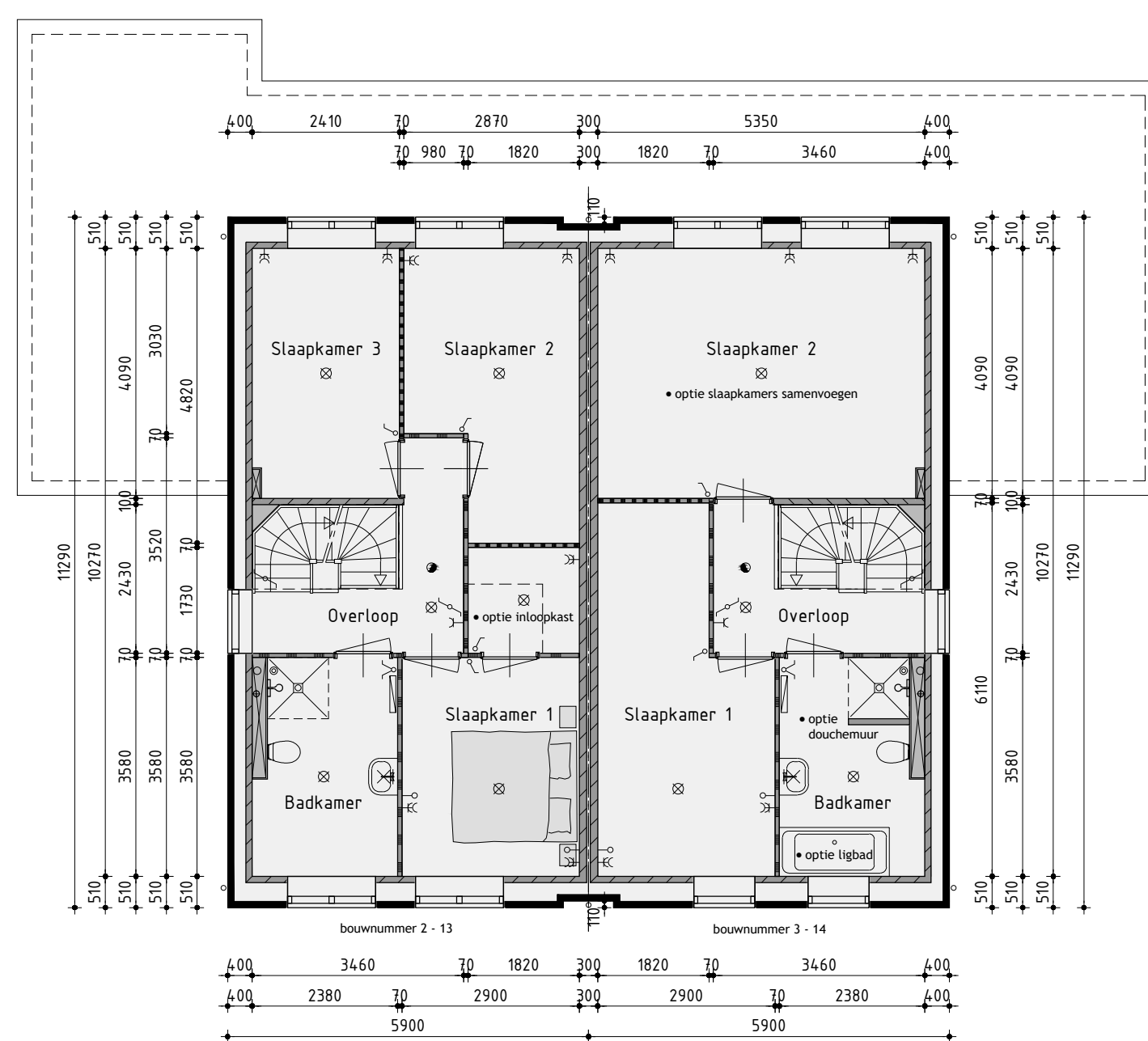
1ste Verdieping
