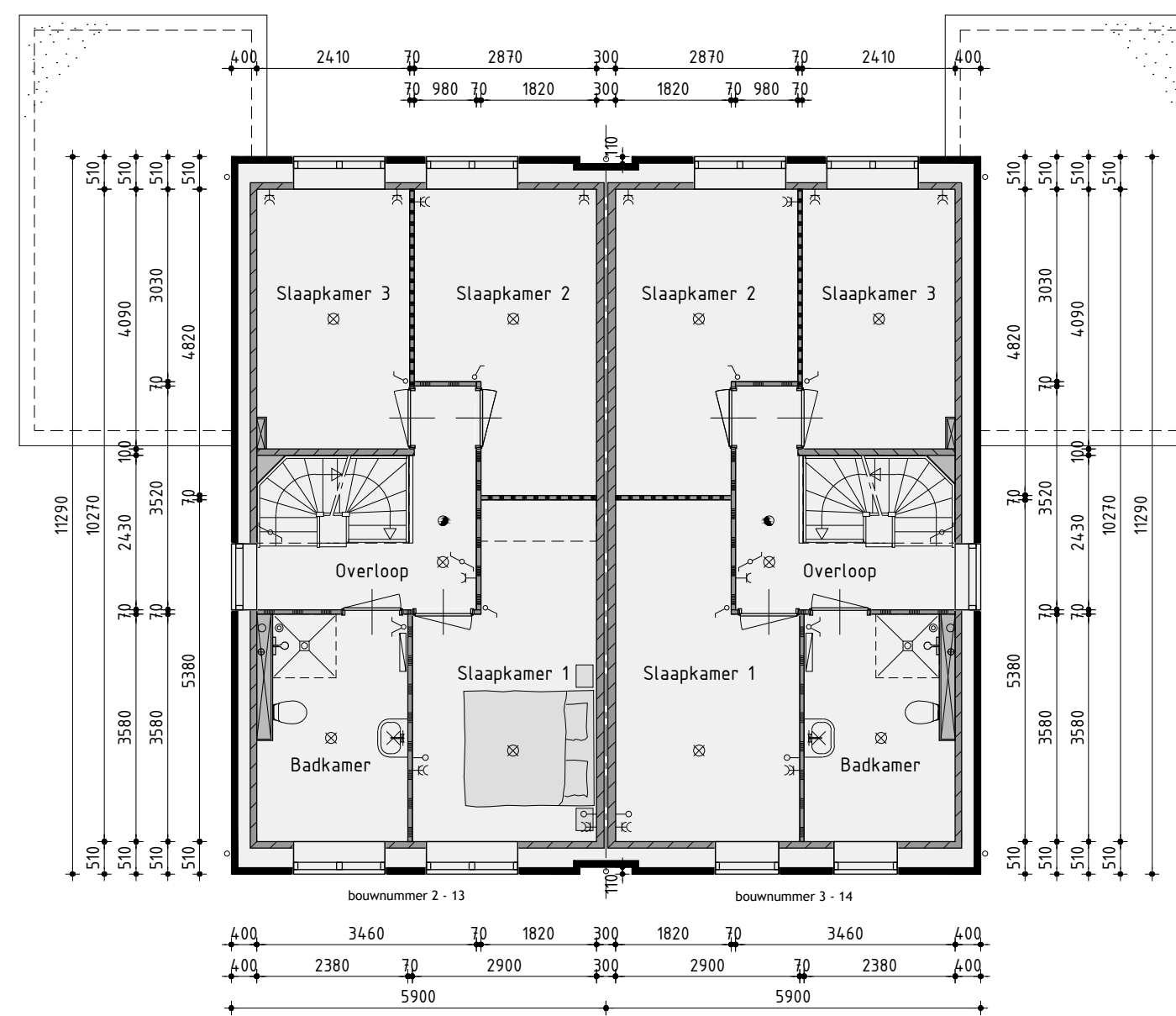
1ste Verdieping
