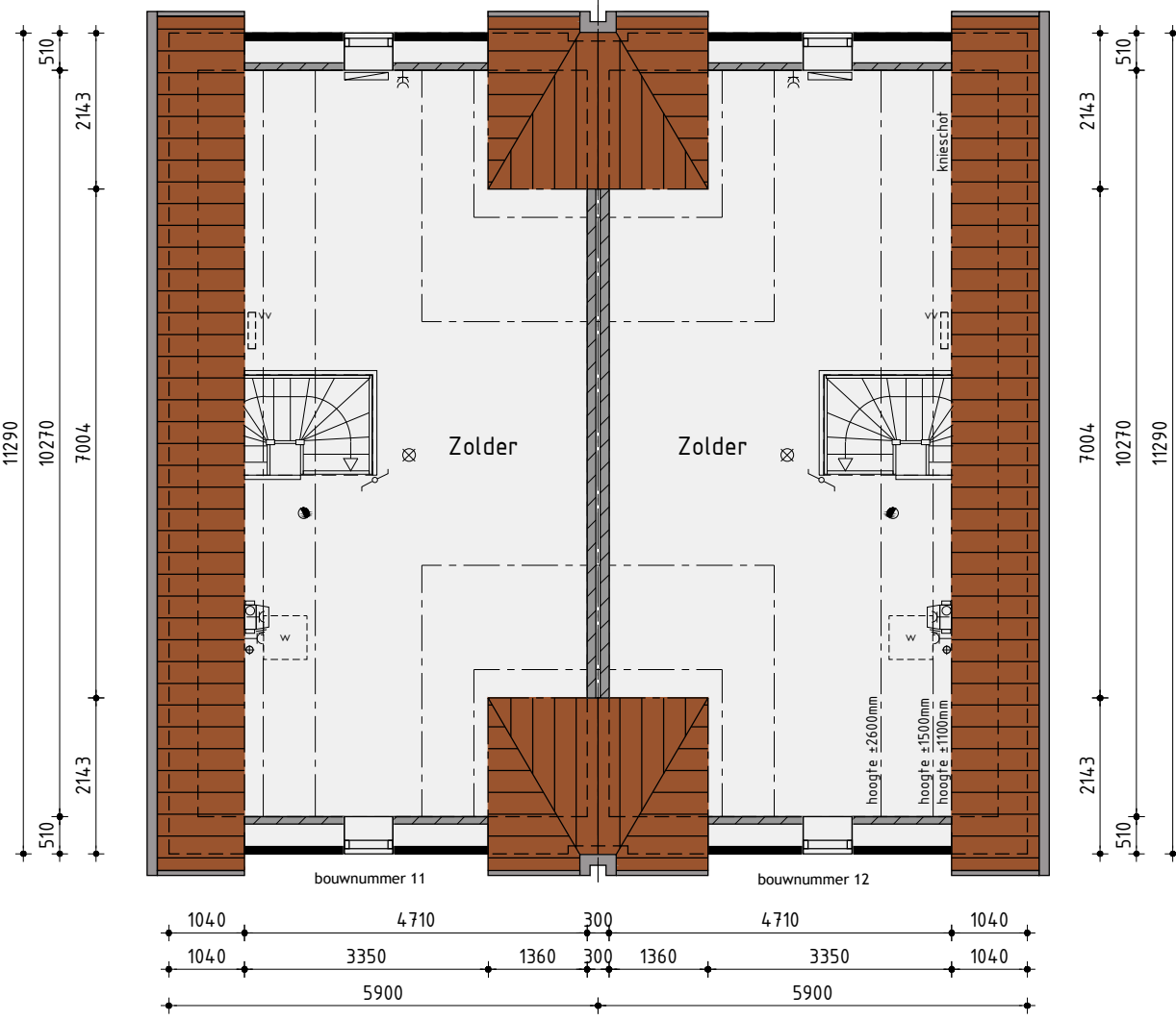
2de Verdieping
