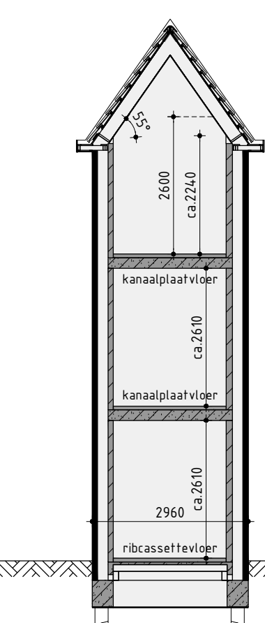
Principe doorsnede C-C
