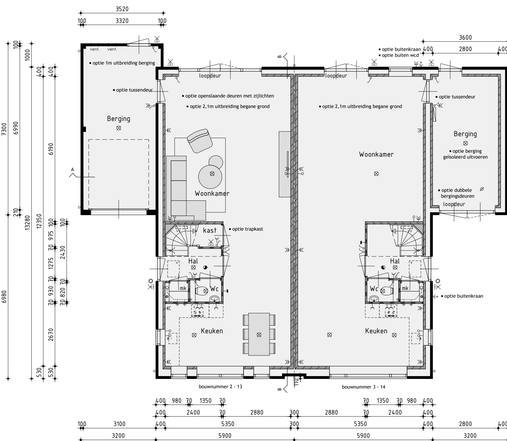
Begane grond
