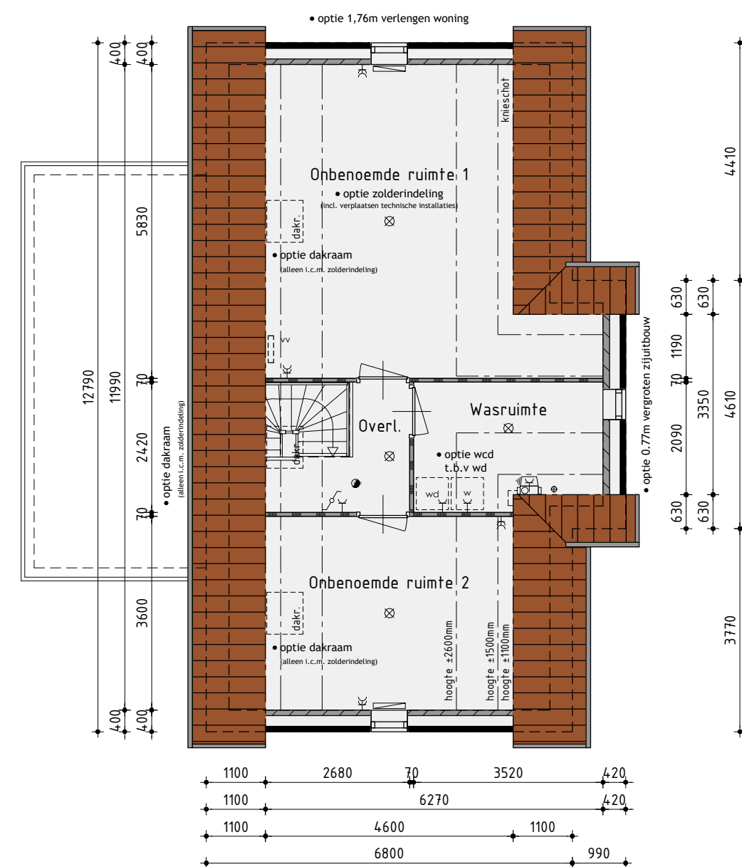
2de Verdieping
