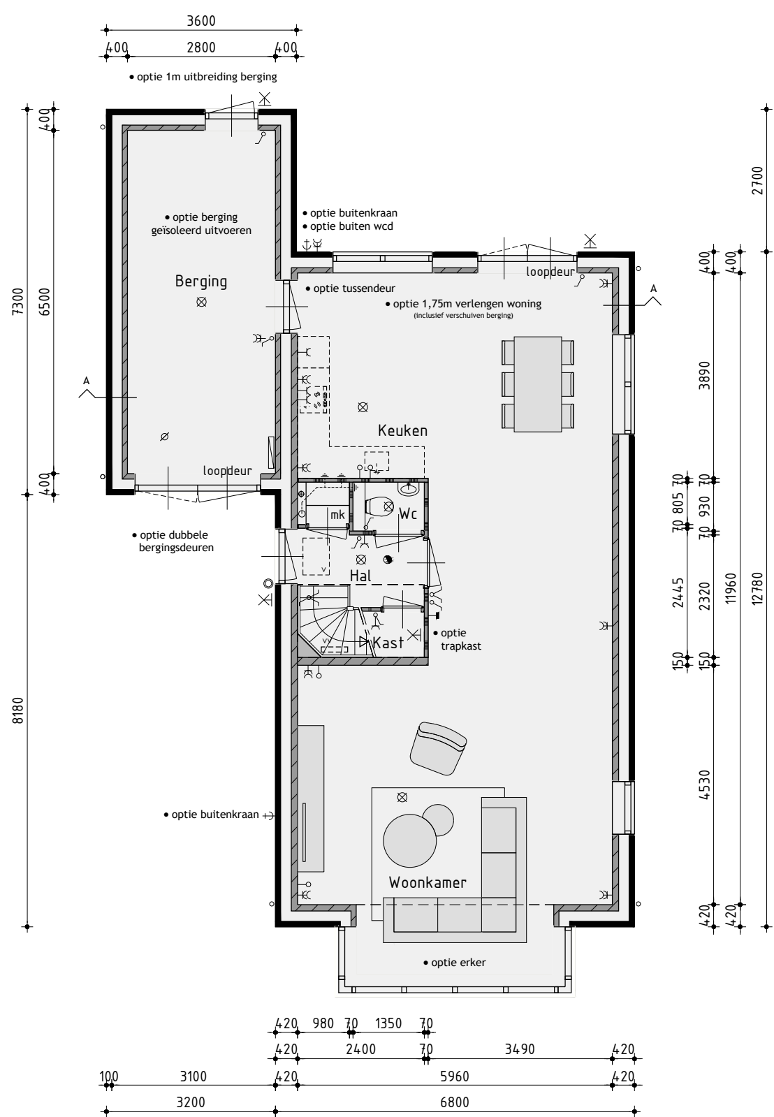
Begane grond v.z.v. vloerverwarming exclusief berging
