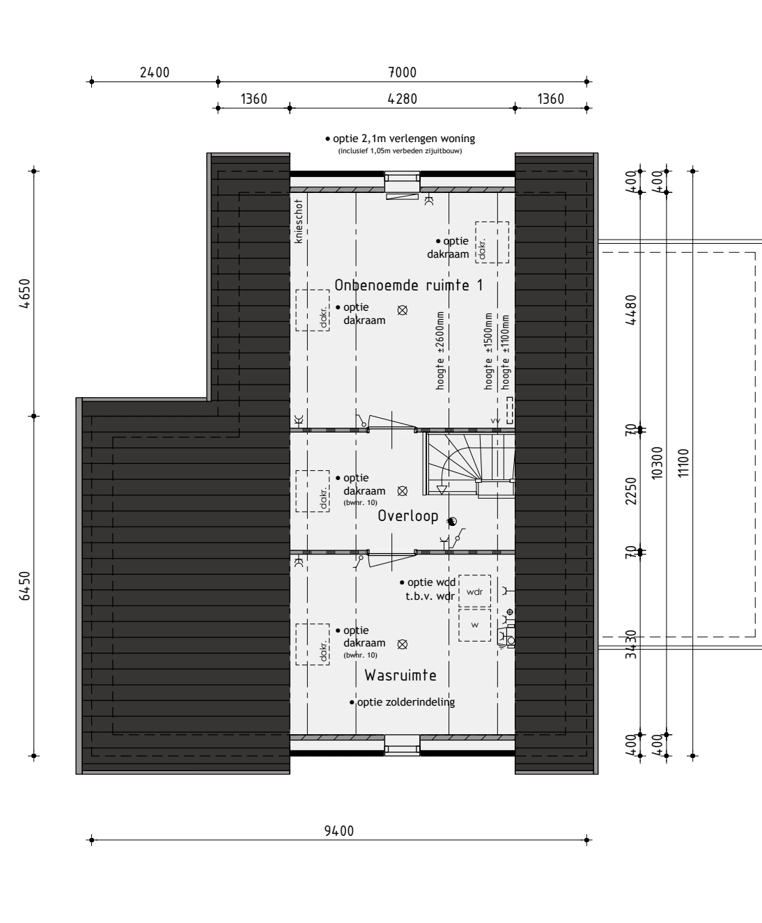
2de Verdieping
