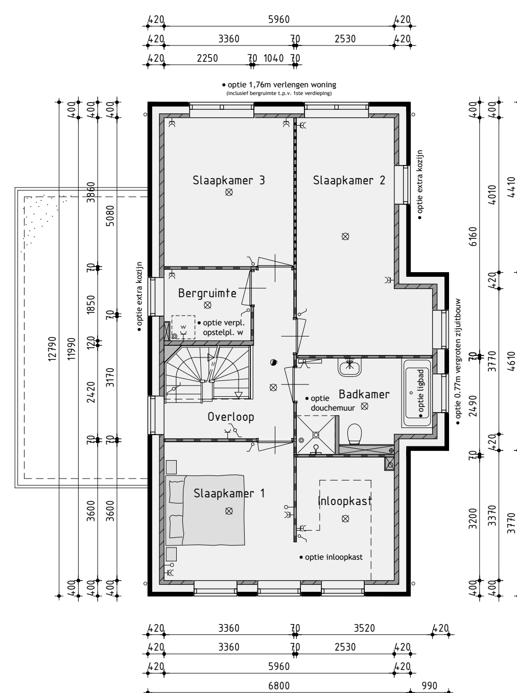
1ste Verdieping
