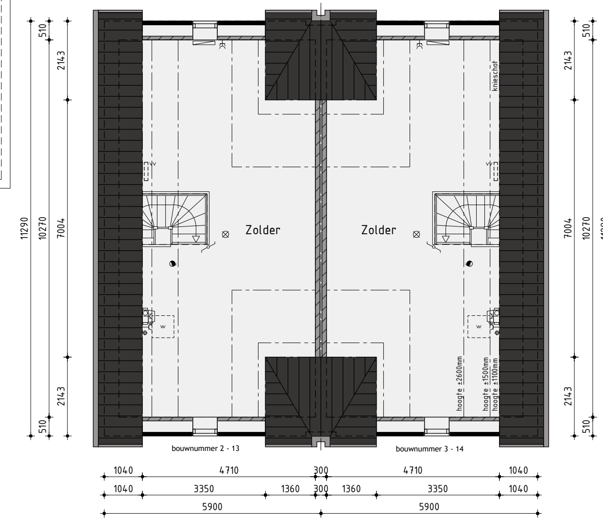
2de Verdieping
