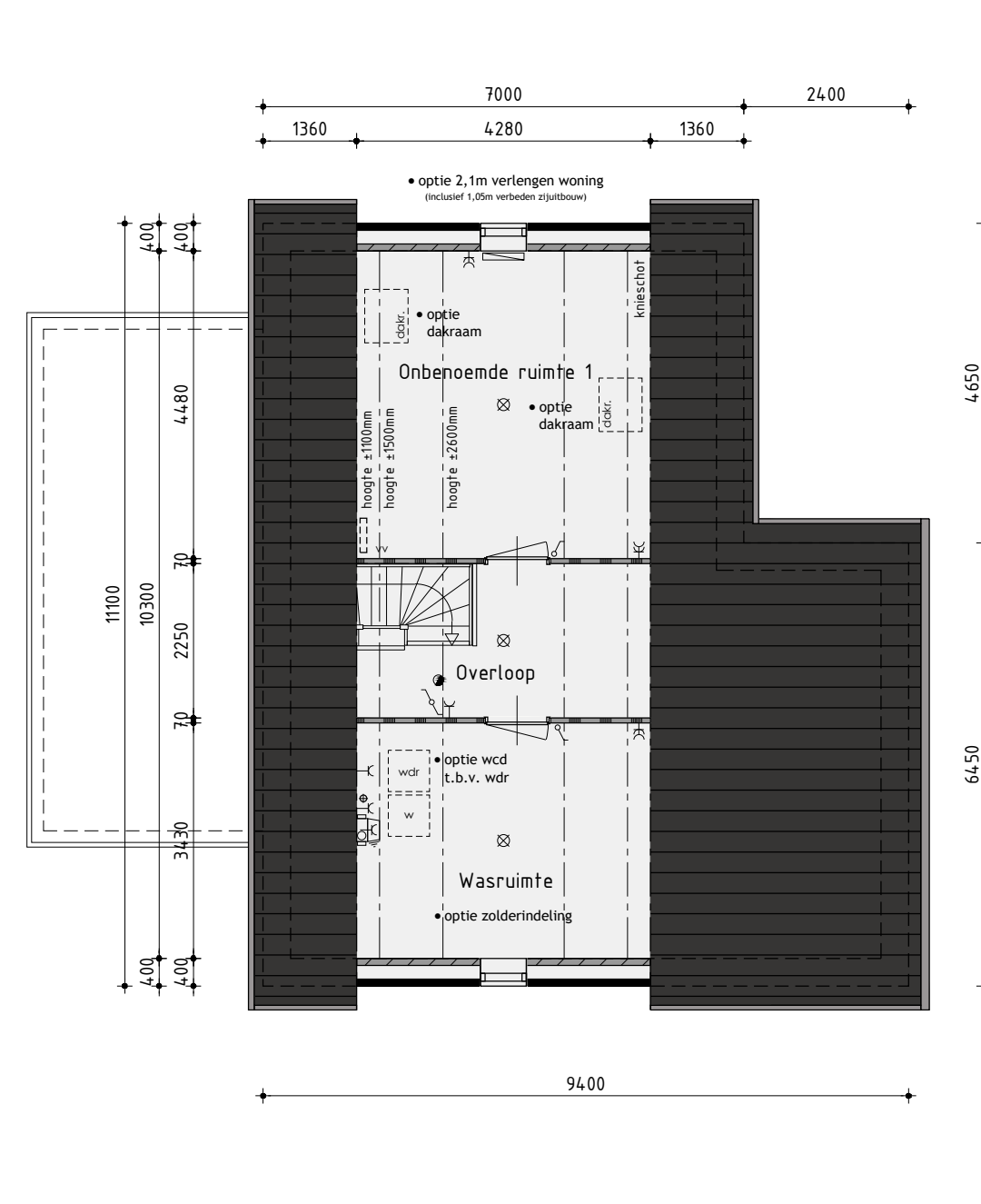
2de Verdieping
