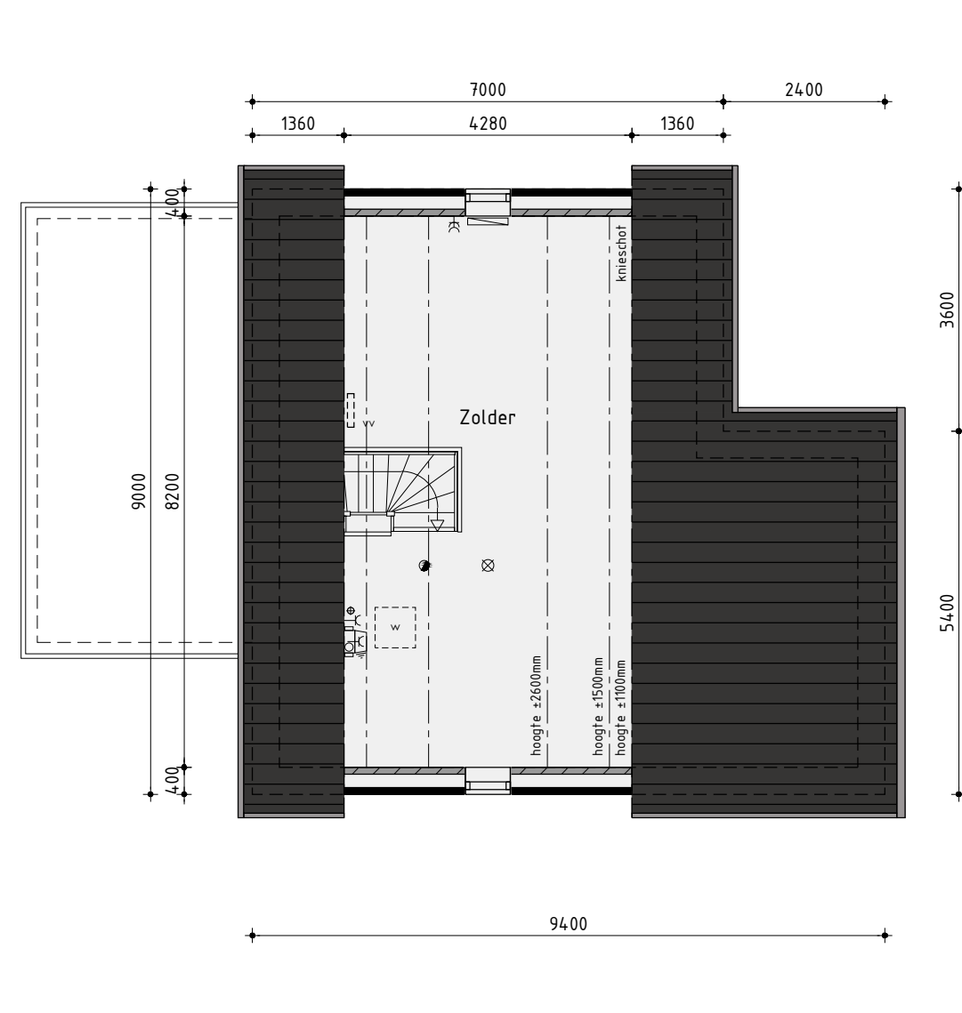
2de Verdieping
