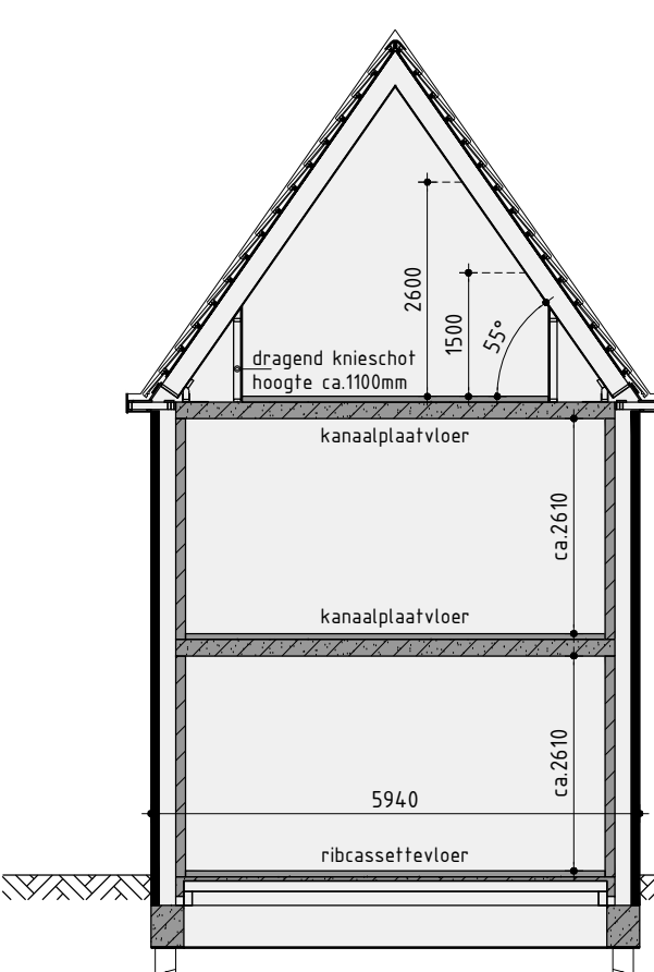
Principe doorsnede B-B
