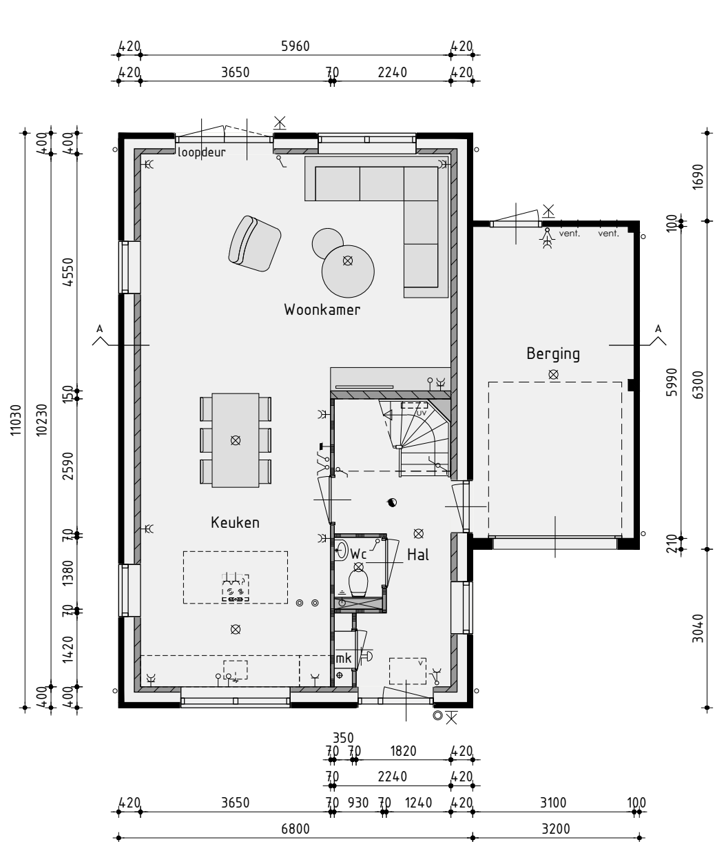
Begane grond
