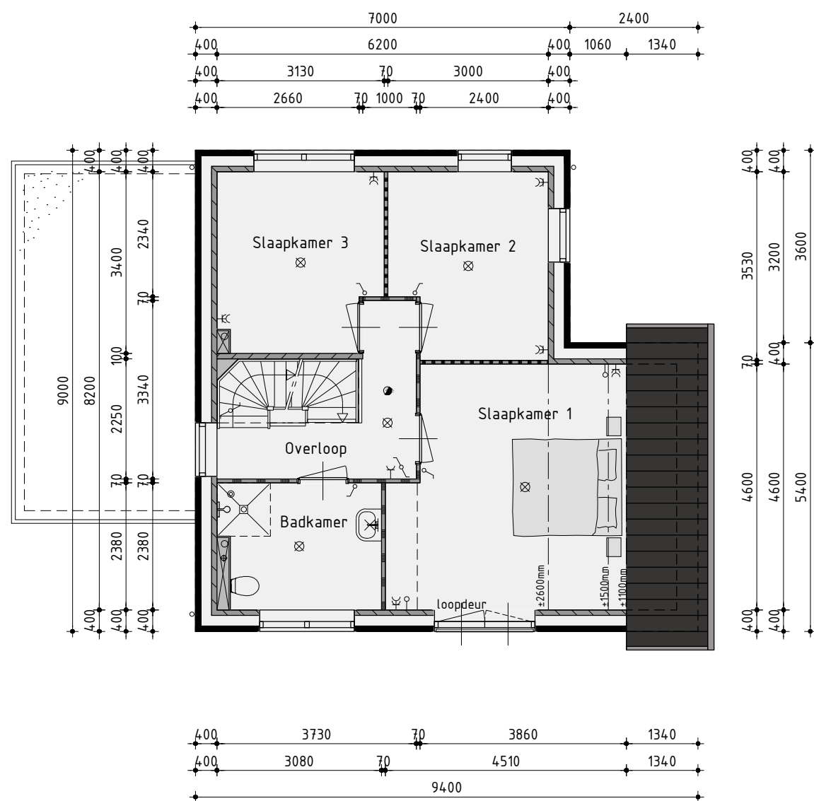
1ste Verdieping
