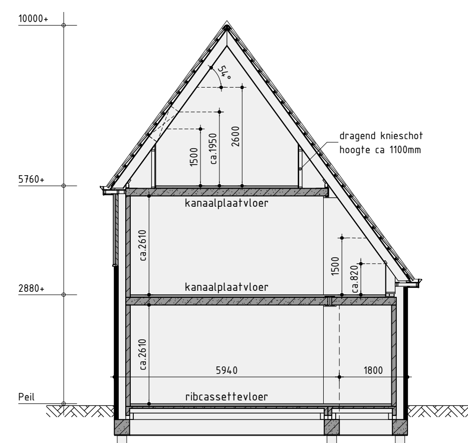
Principe doorsnede B-B
