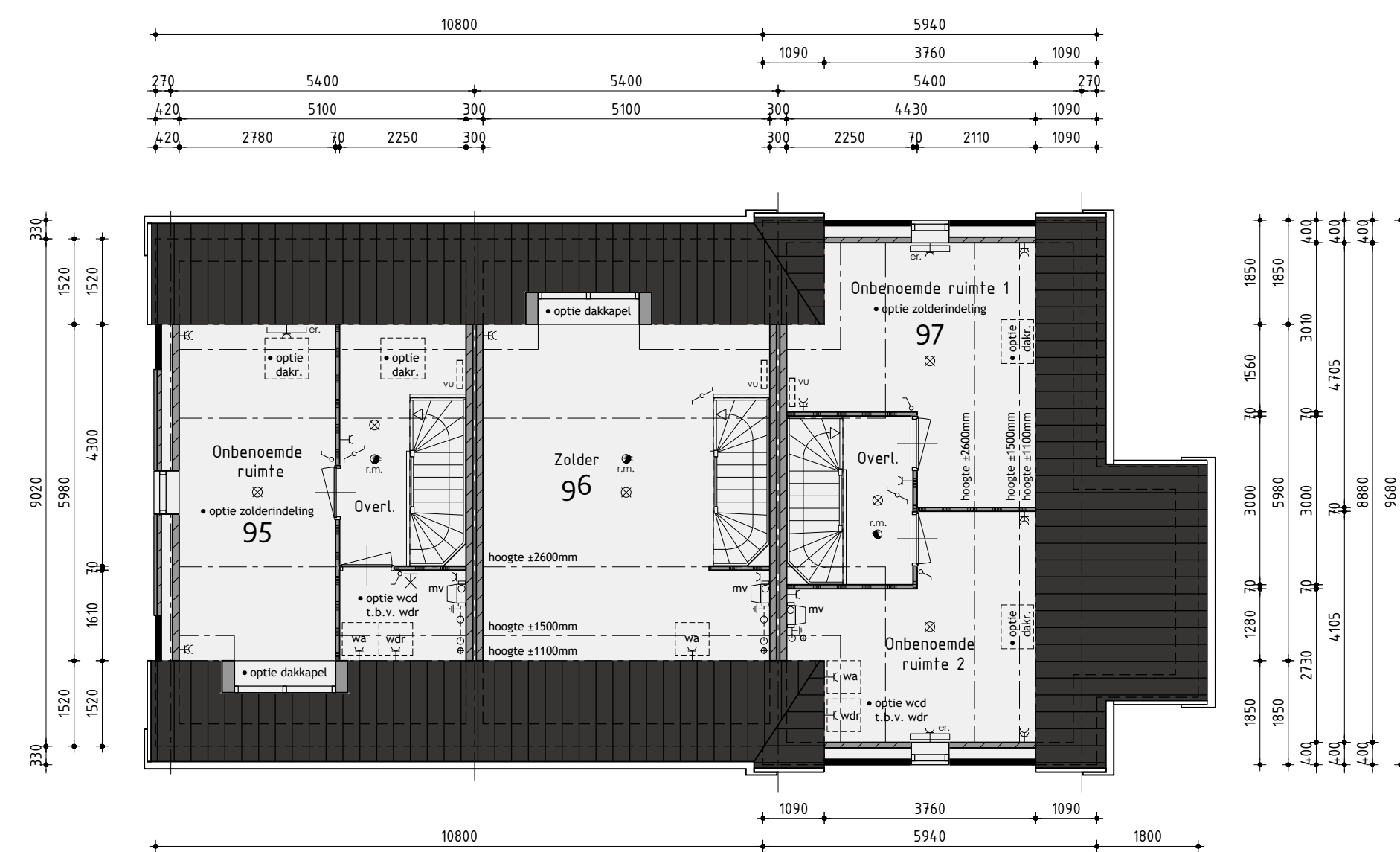
2de Verdieping
