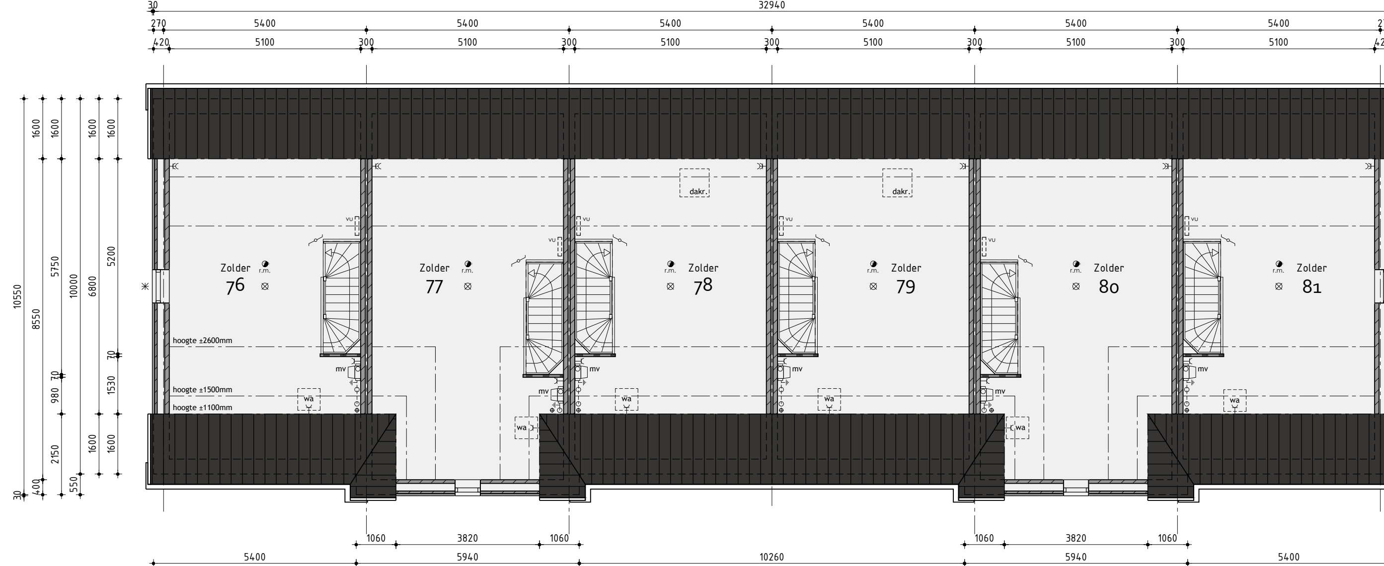
2de Verdieping
