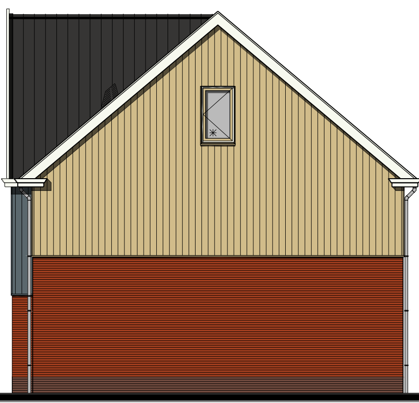
Rechter zijgevel
