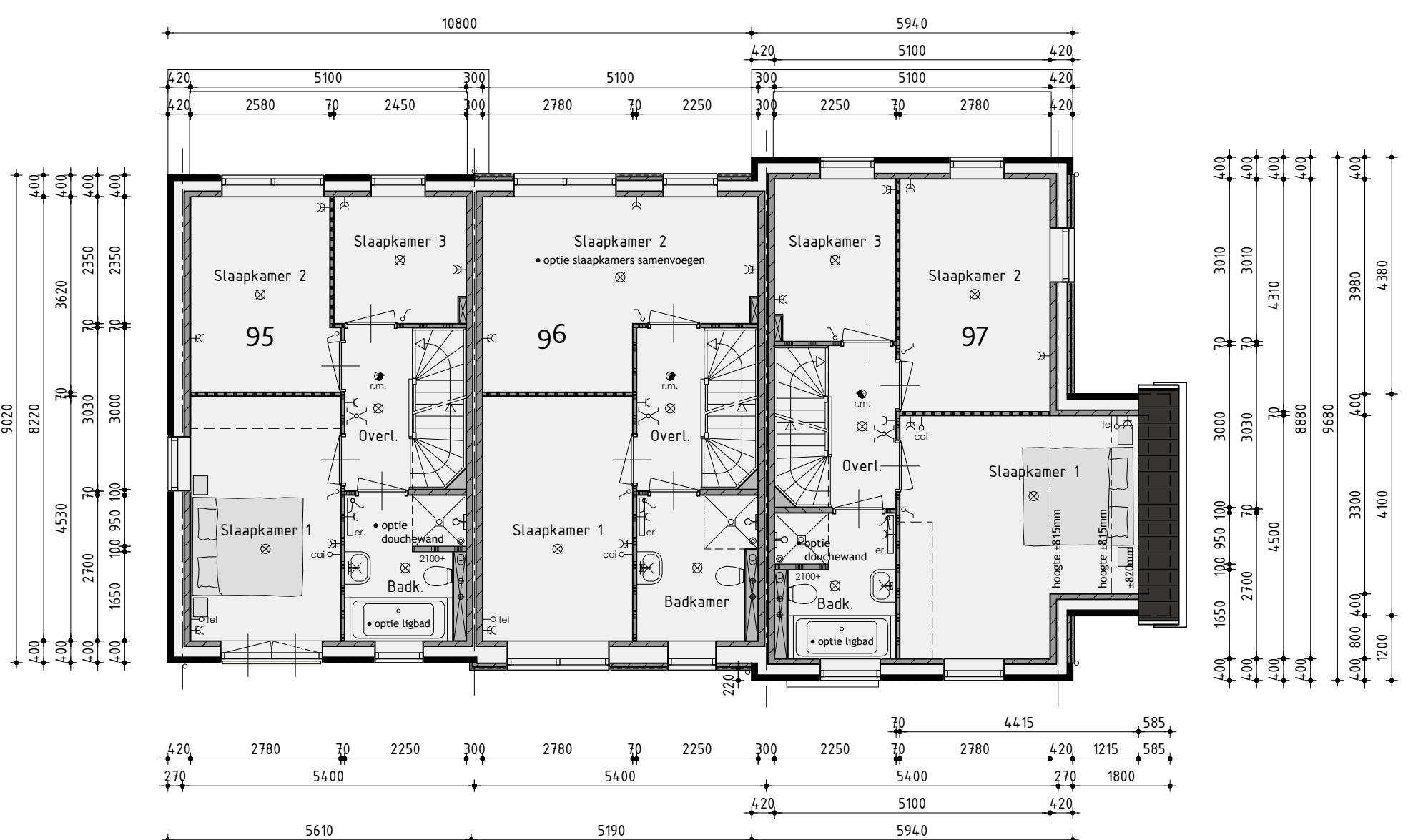
1ste Verdieping
