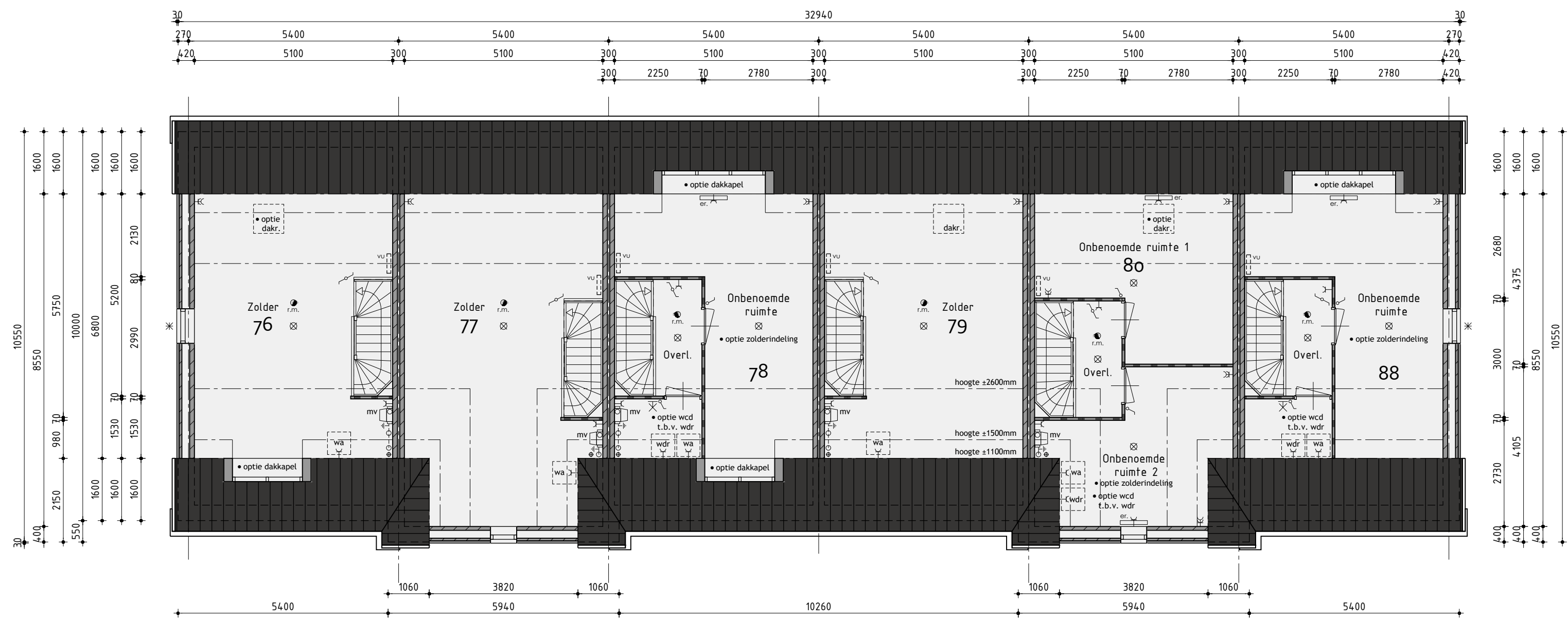
2de Verdieping
