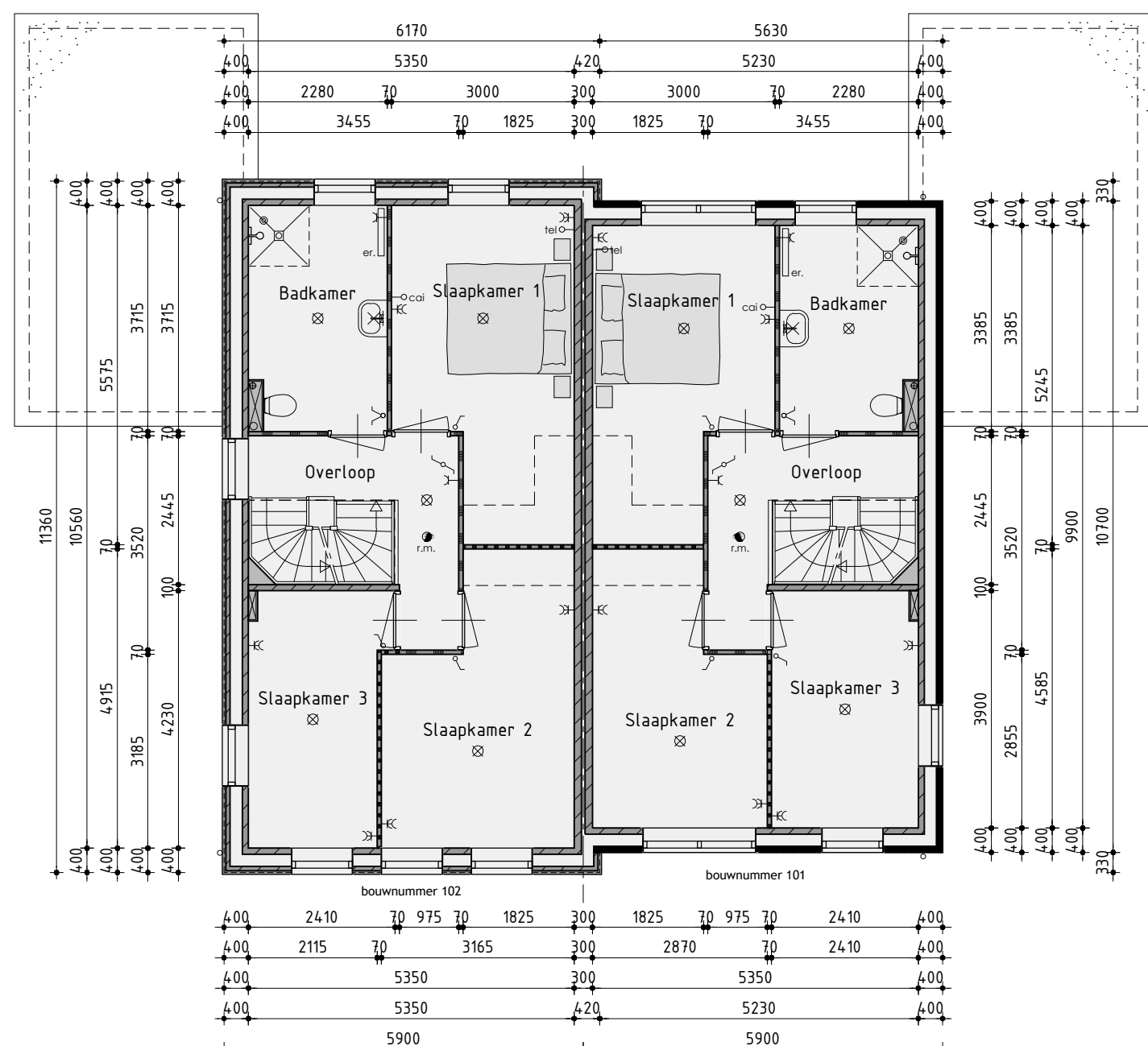
1ste Verdieping
