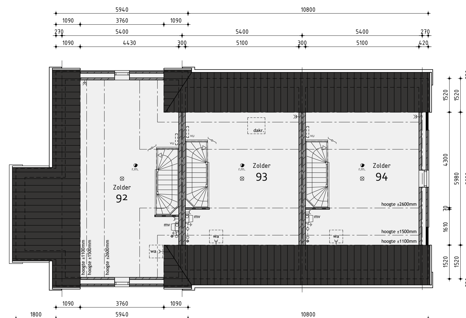
2de Verdieping
