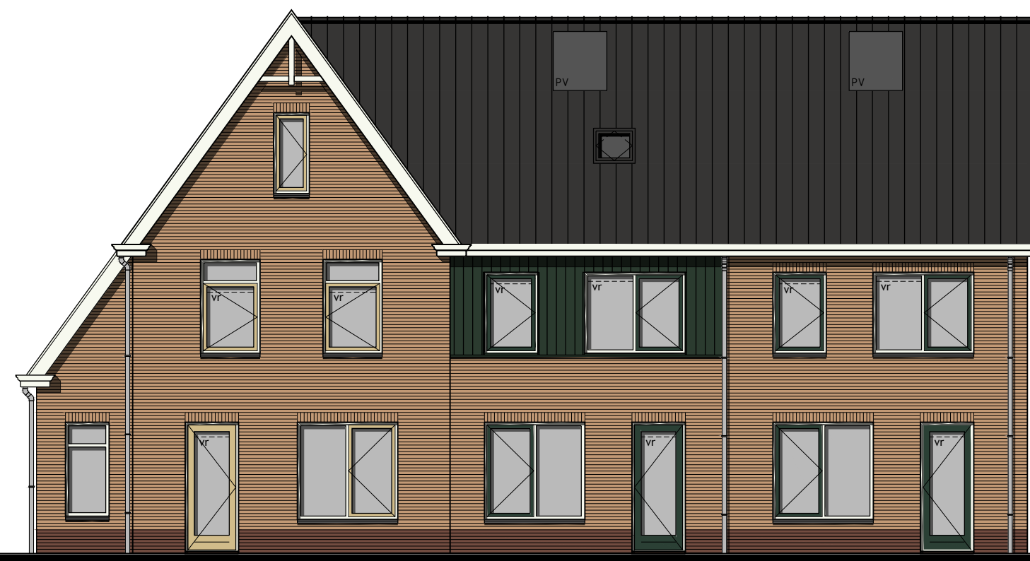
Achtergevel
