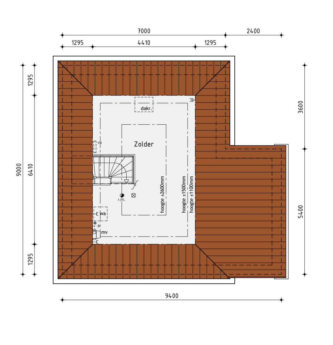
2de Verdieping
