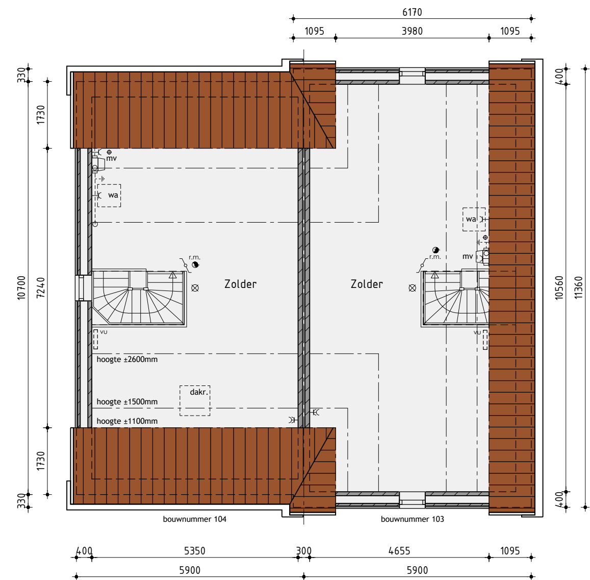
2de Verdieping
