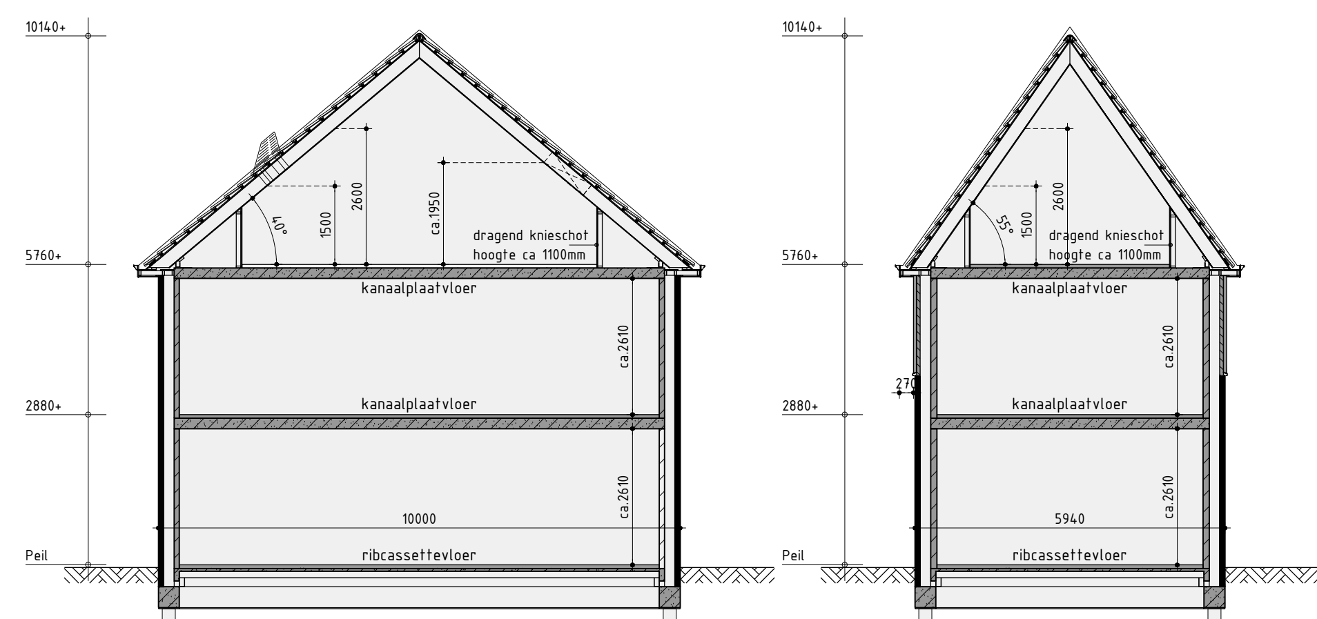
Principe doorsnede A-A
