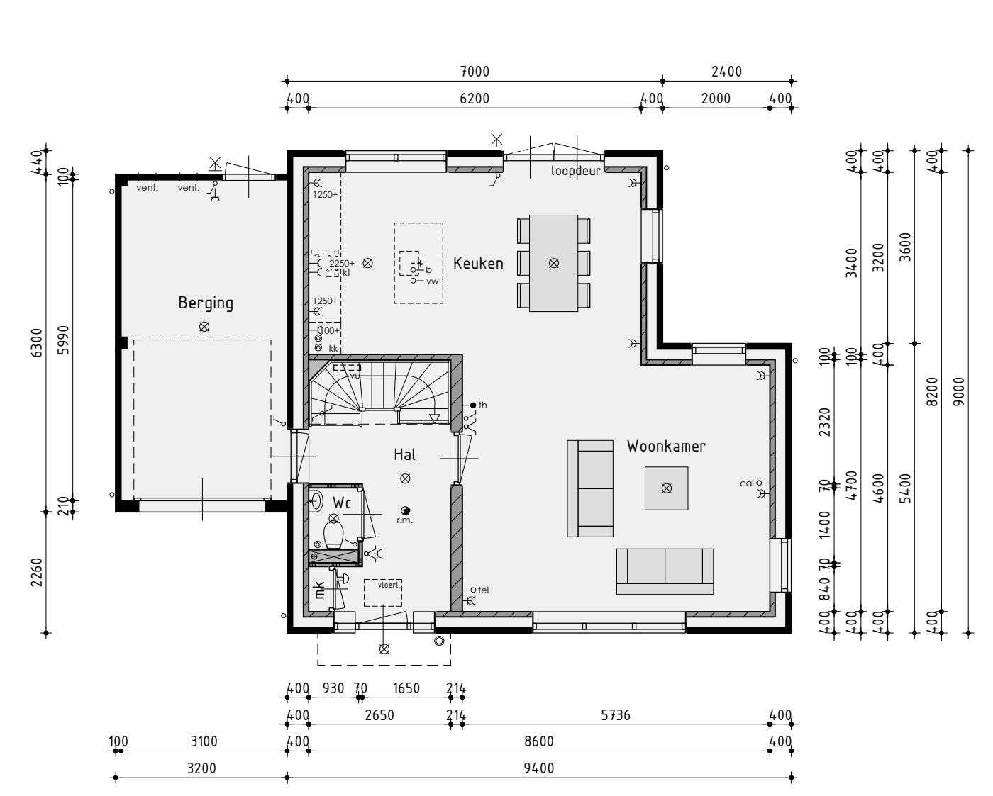
Begane grond v.z.v. vloerverwarming excl. berging
