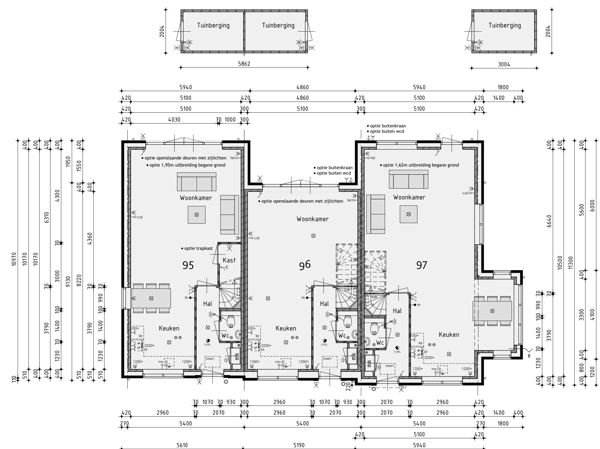
Begane grond
