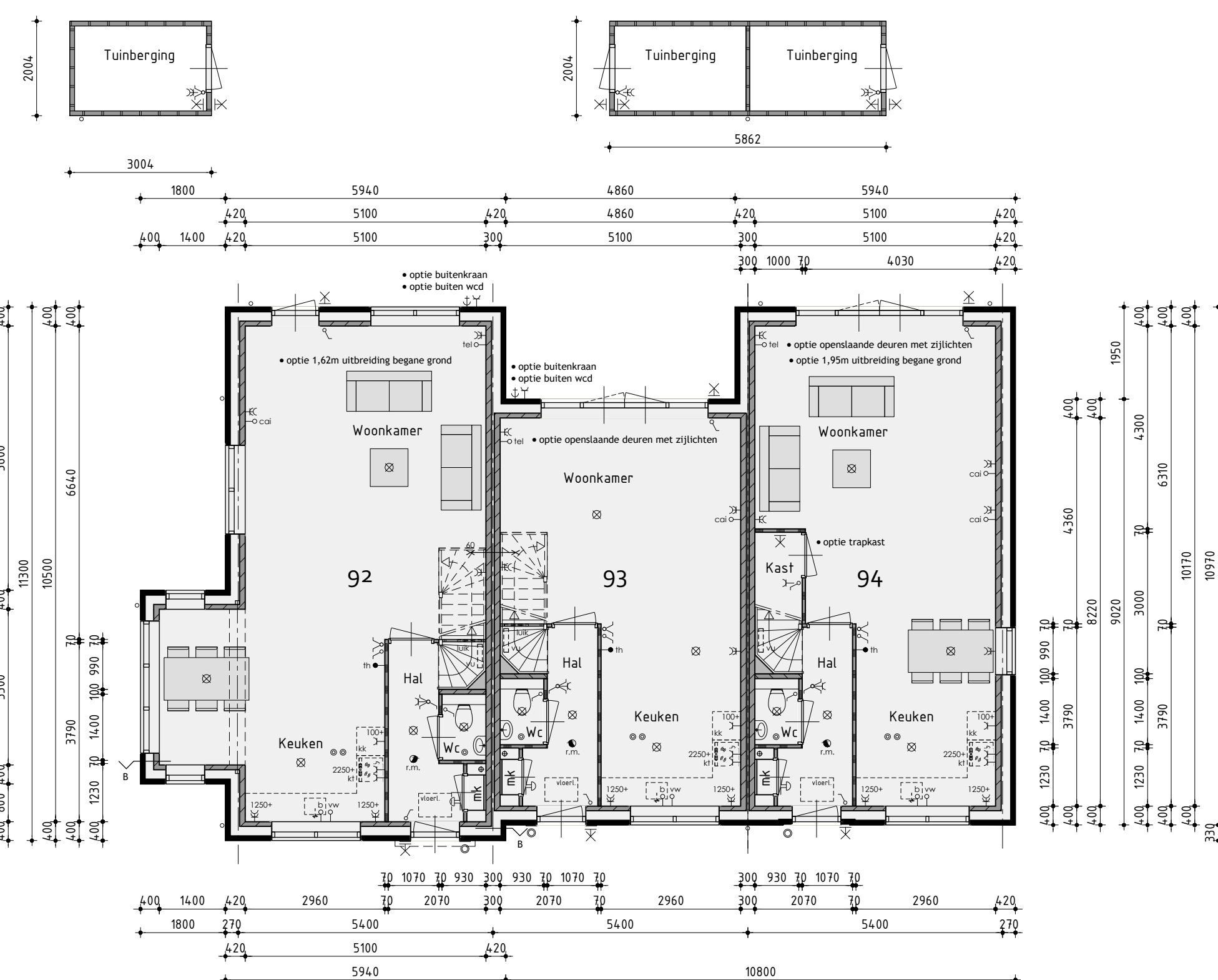
Begane grond
