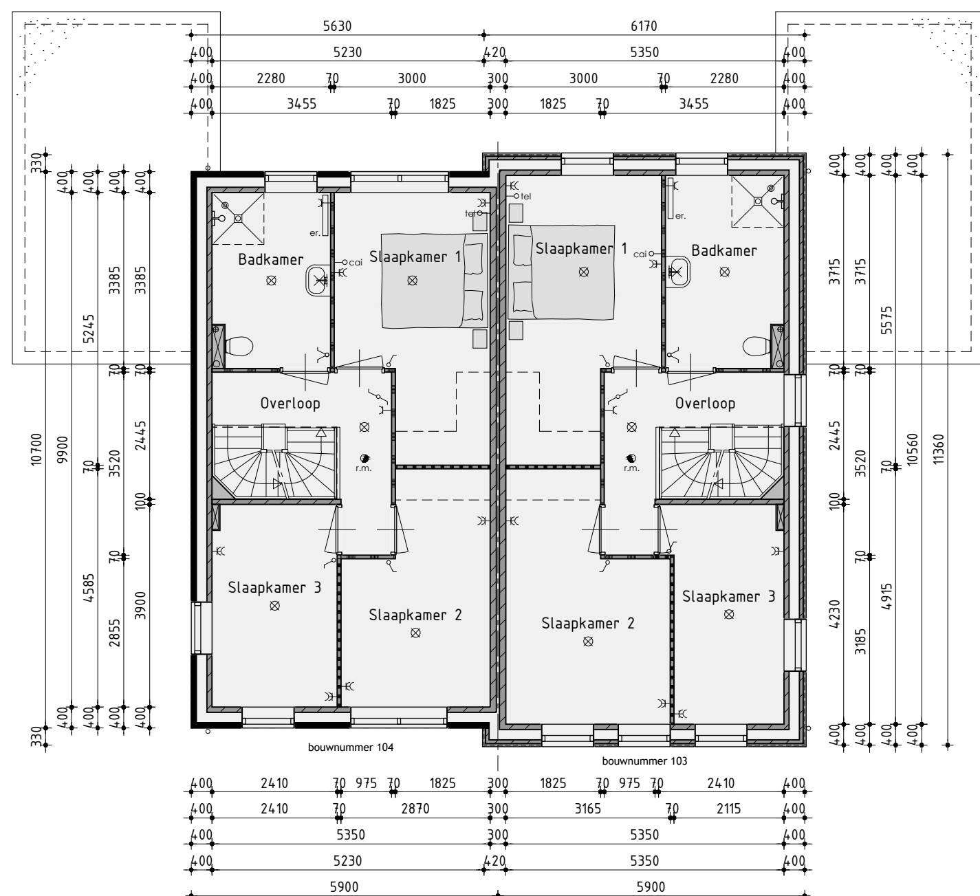
1ste Verdieping
