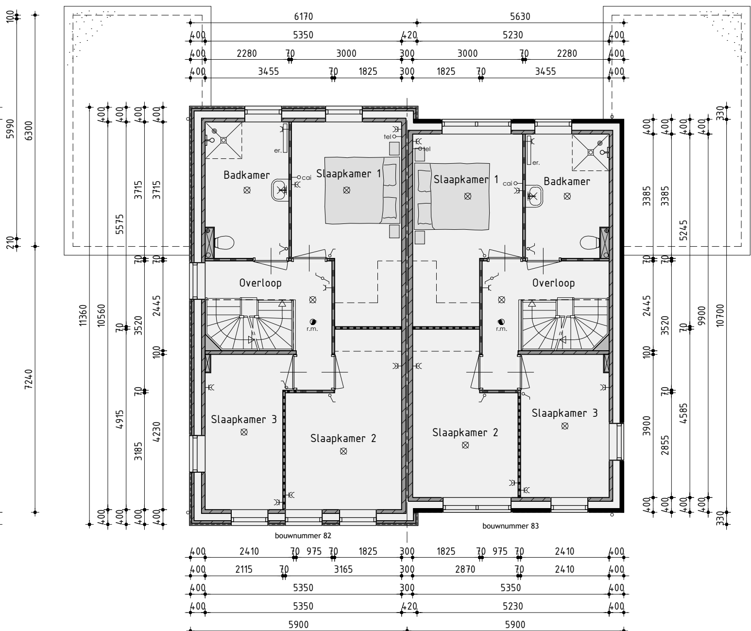
1ste Verdieping
