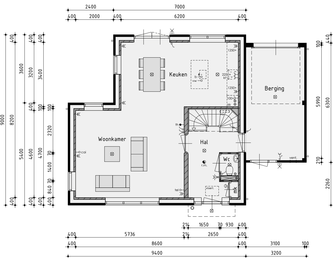
Begane grond
