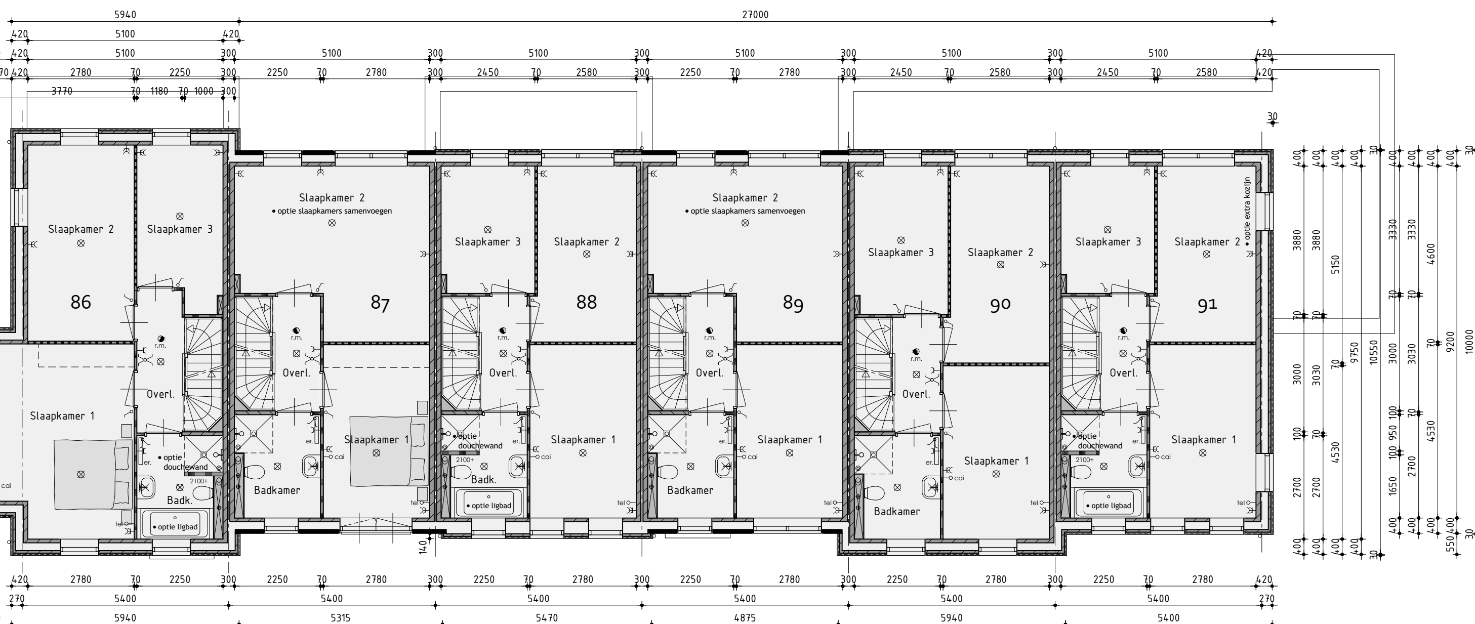
1ste Verdieping
