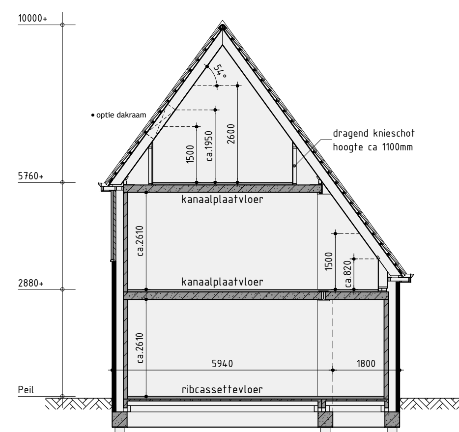
Principe doorsnede B-B
