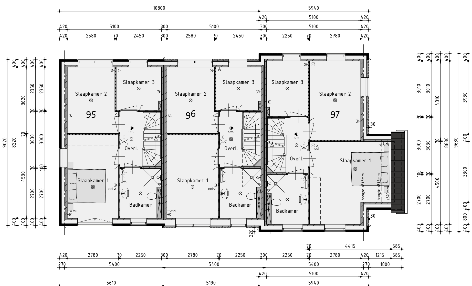
1ste Verdieping v.z.v. vloerverwarming
