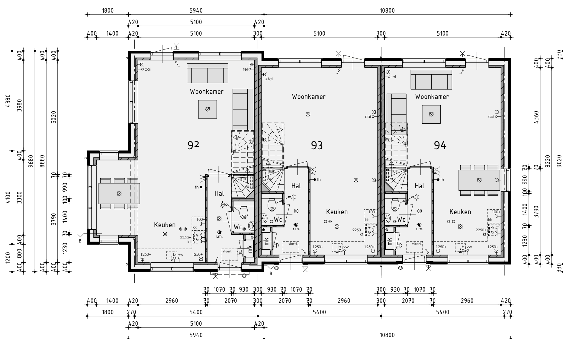
Begane grond
