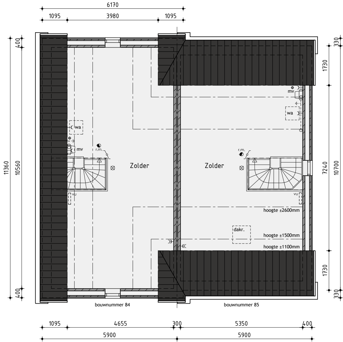
2de Verdieping
