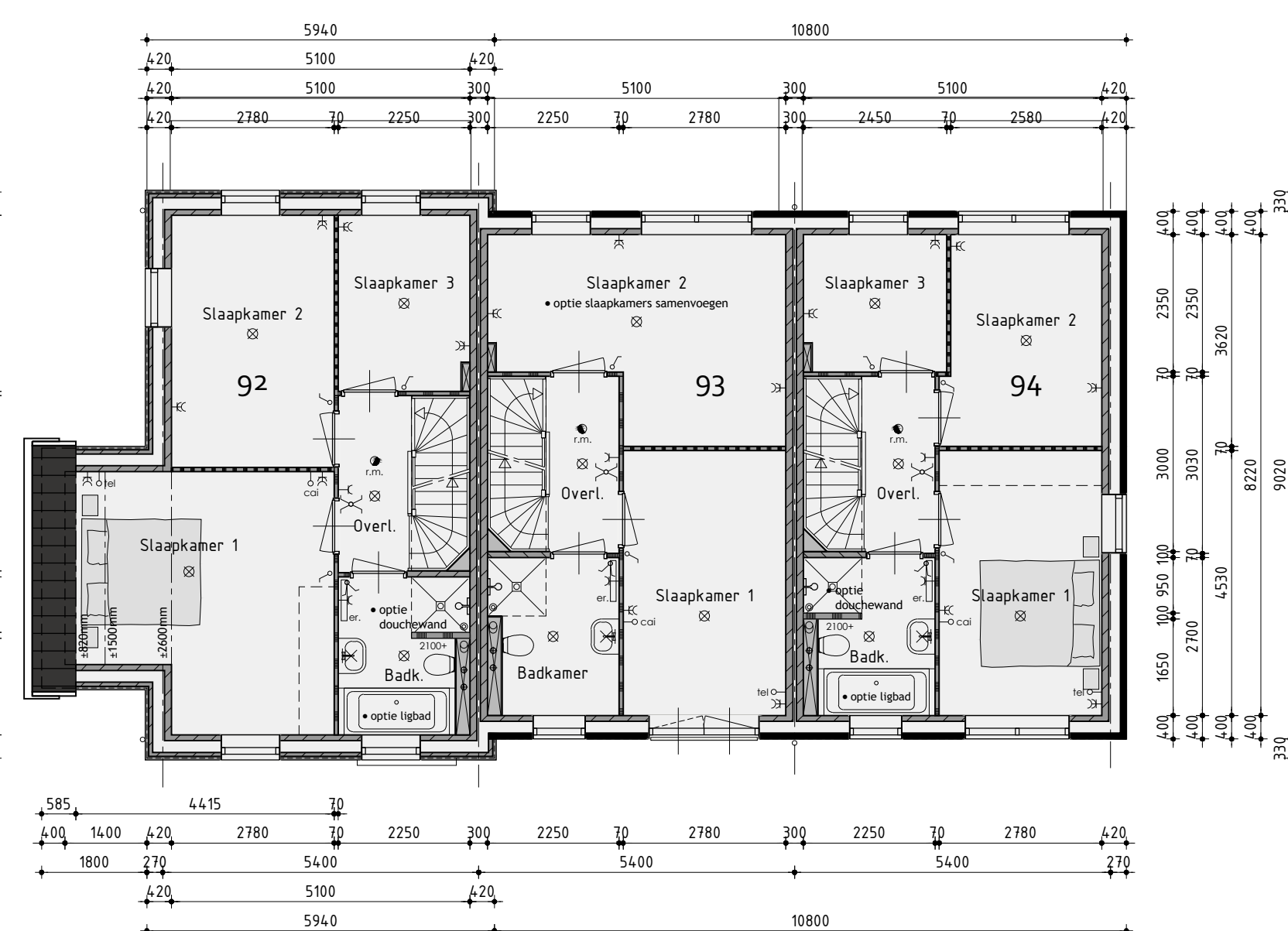
1ste Verdieping
