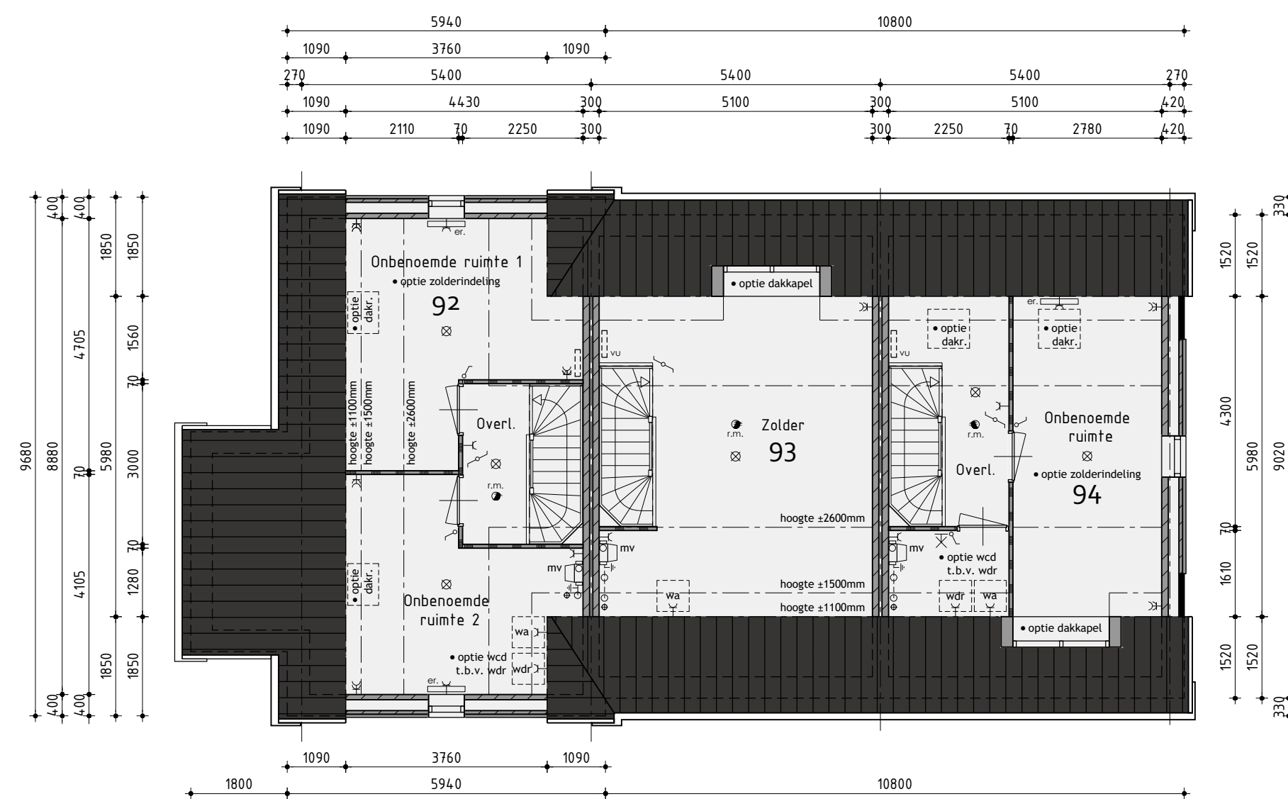
2de Verdieping
