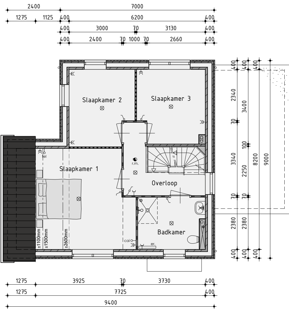
1ste Verdieping
