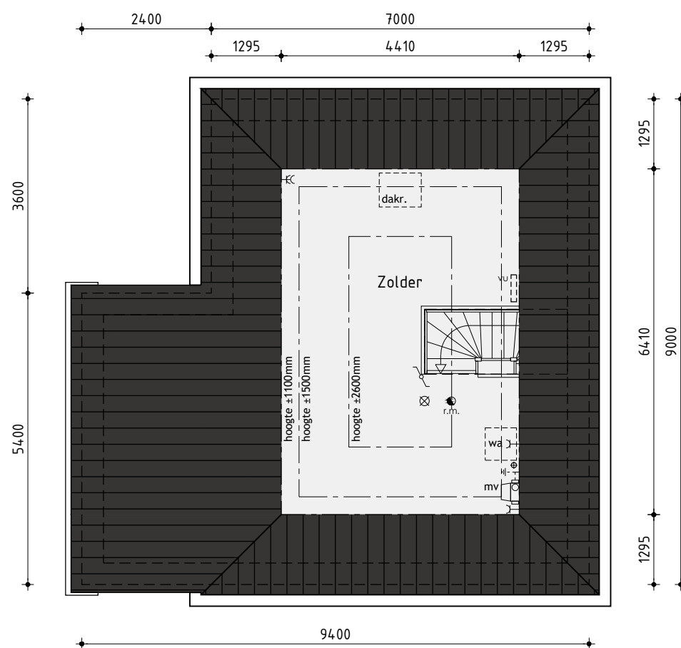
2de Verdieping
