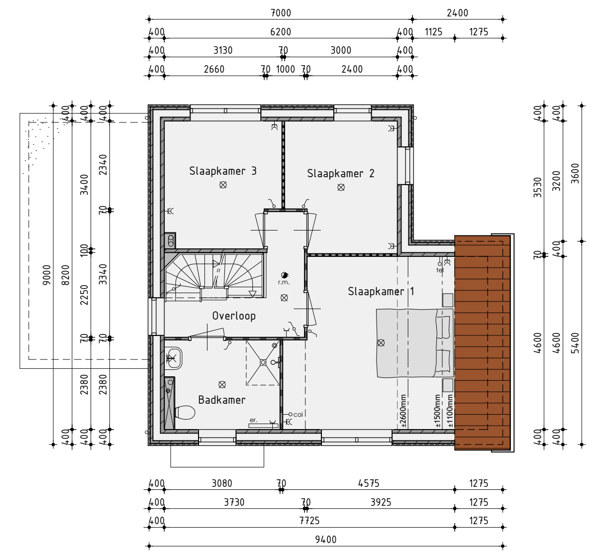
1ste Verdieping v.z.v. vloerverwarming
