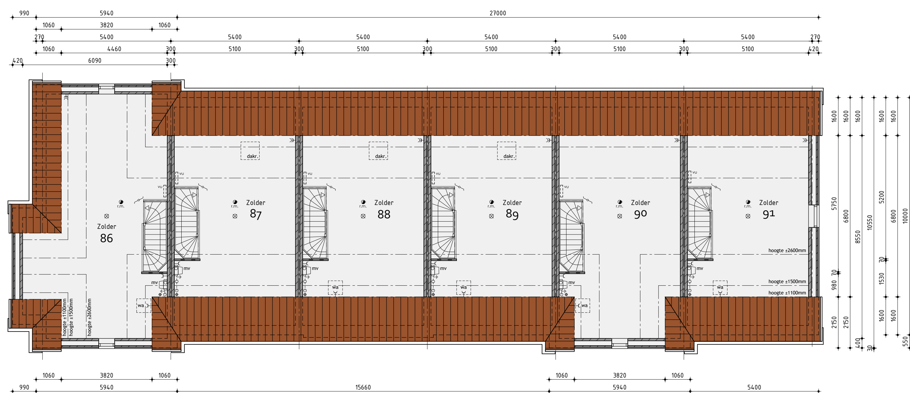
2de Verdieping
