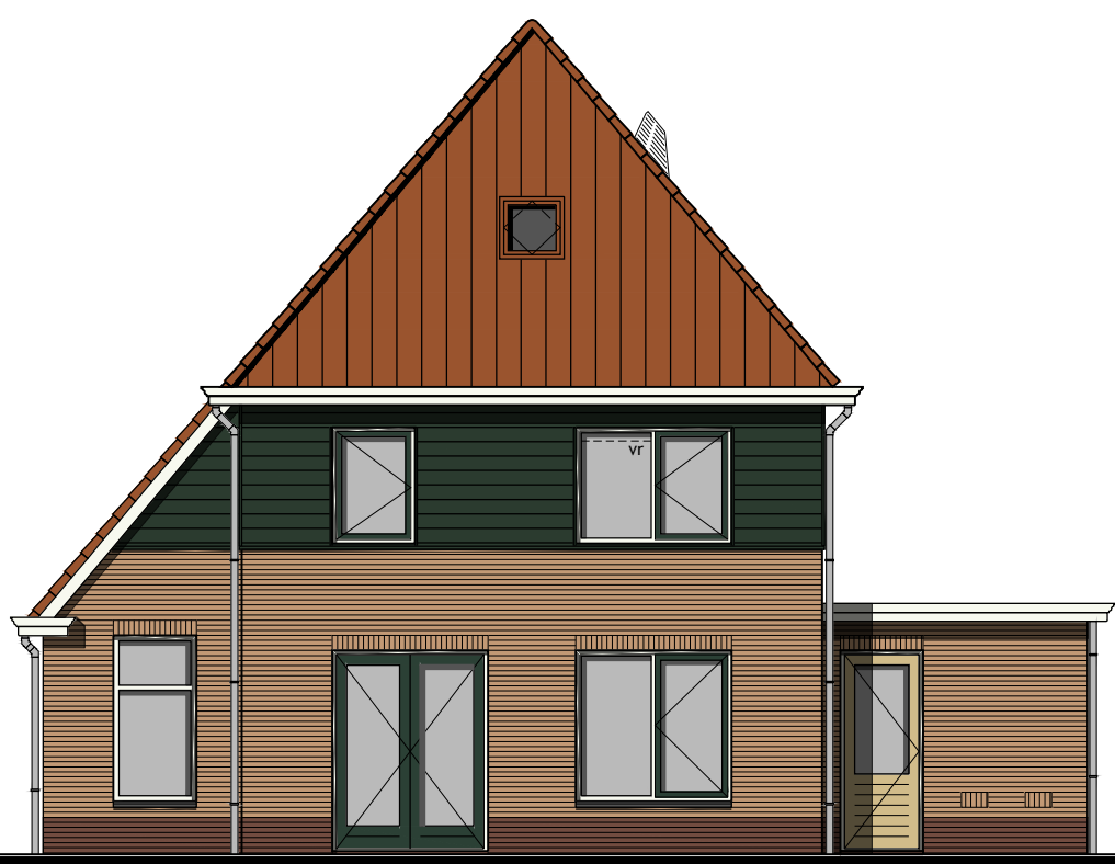
Achtergevel
