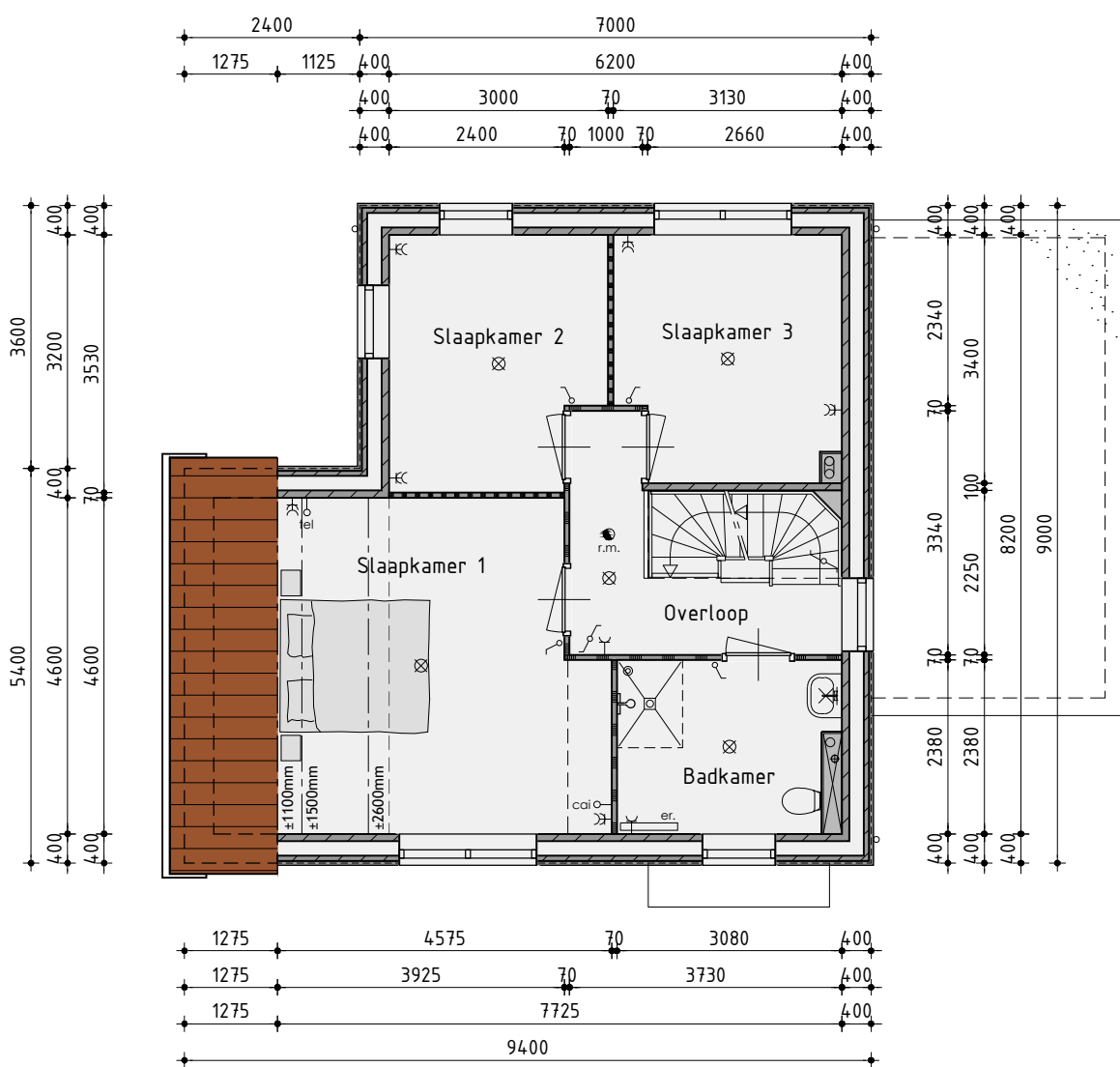
1ste Verdieping
