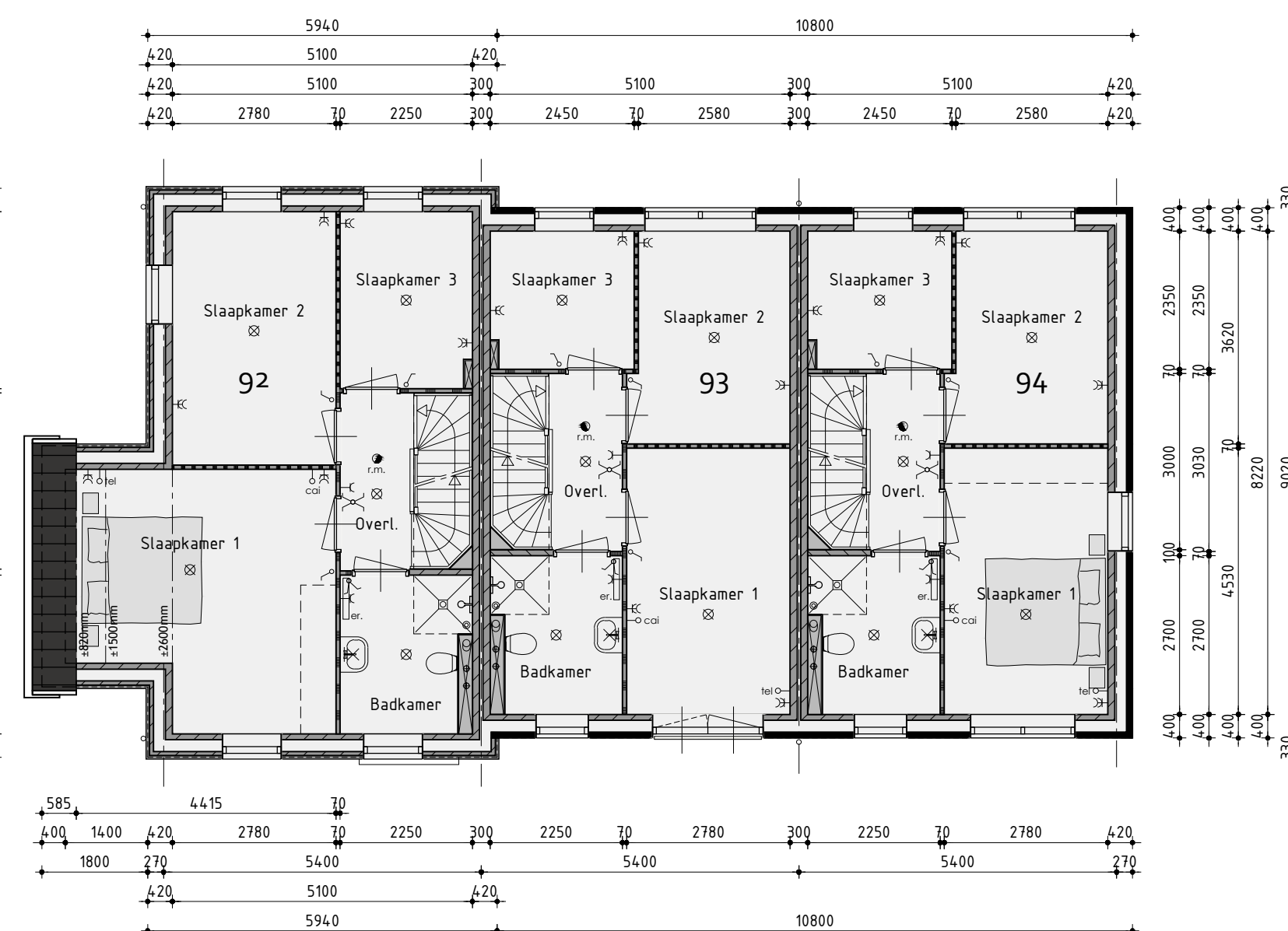
1ste Verdieping
