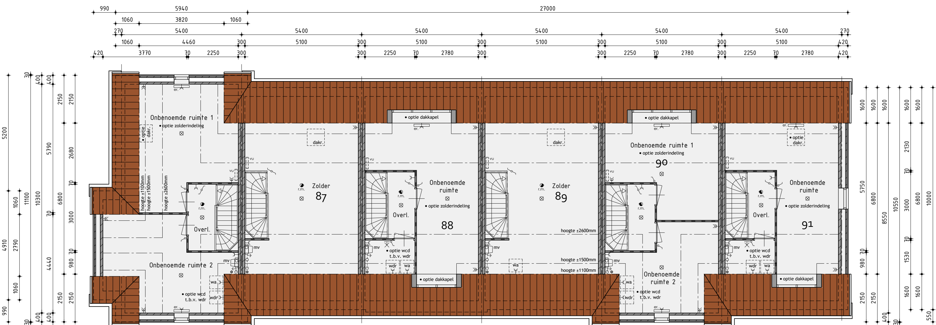
2de Verdieping
