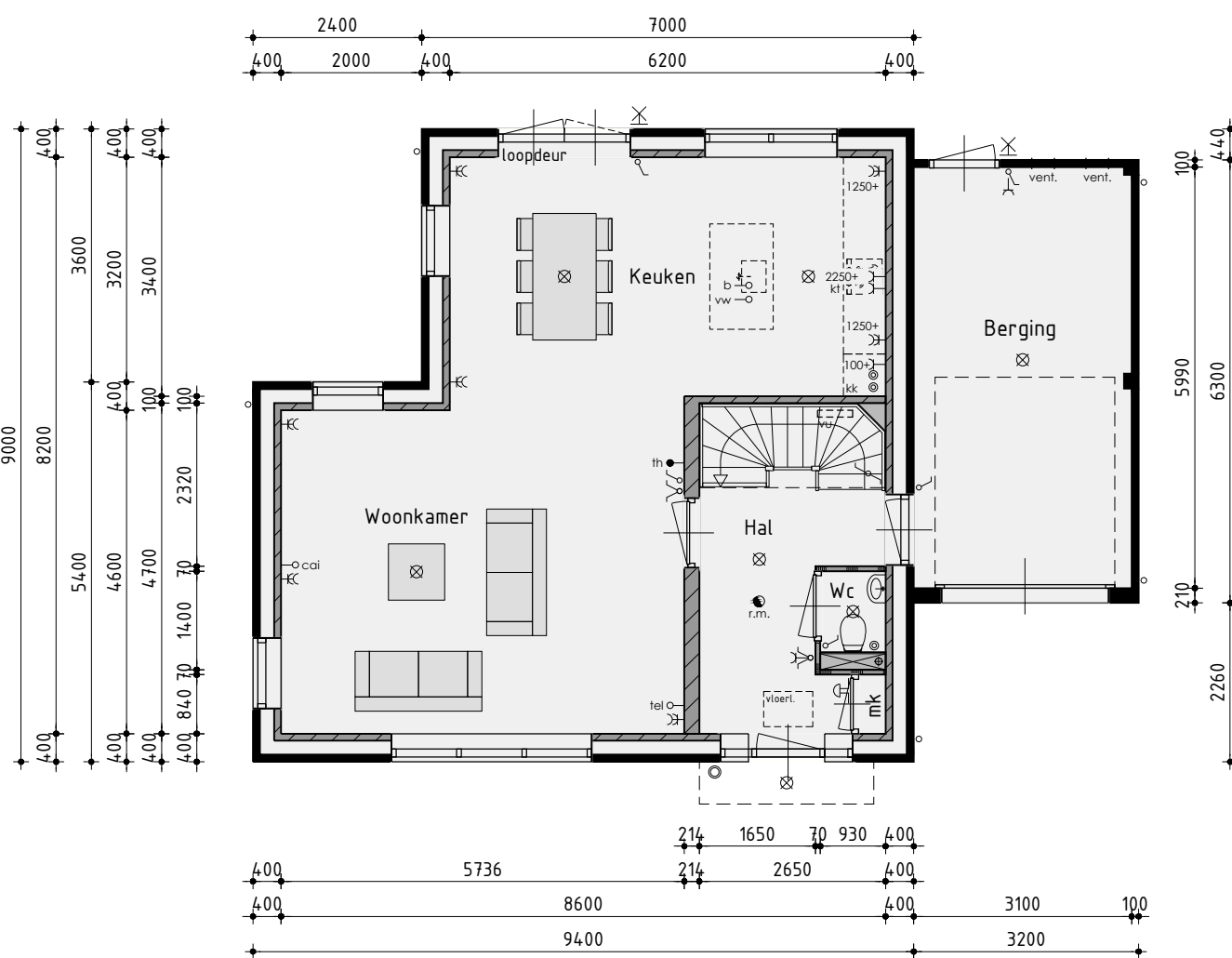
Begane grond
