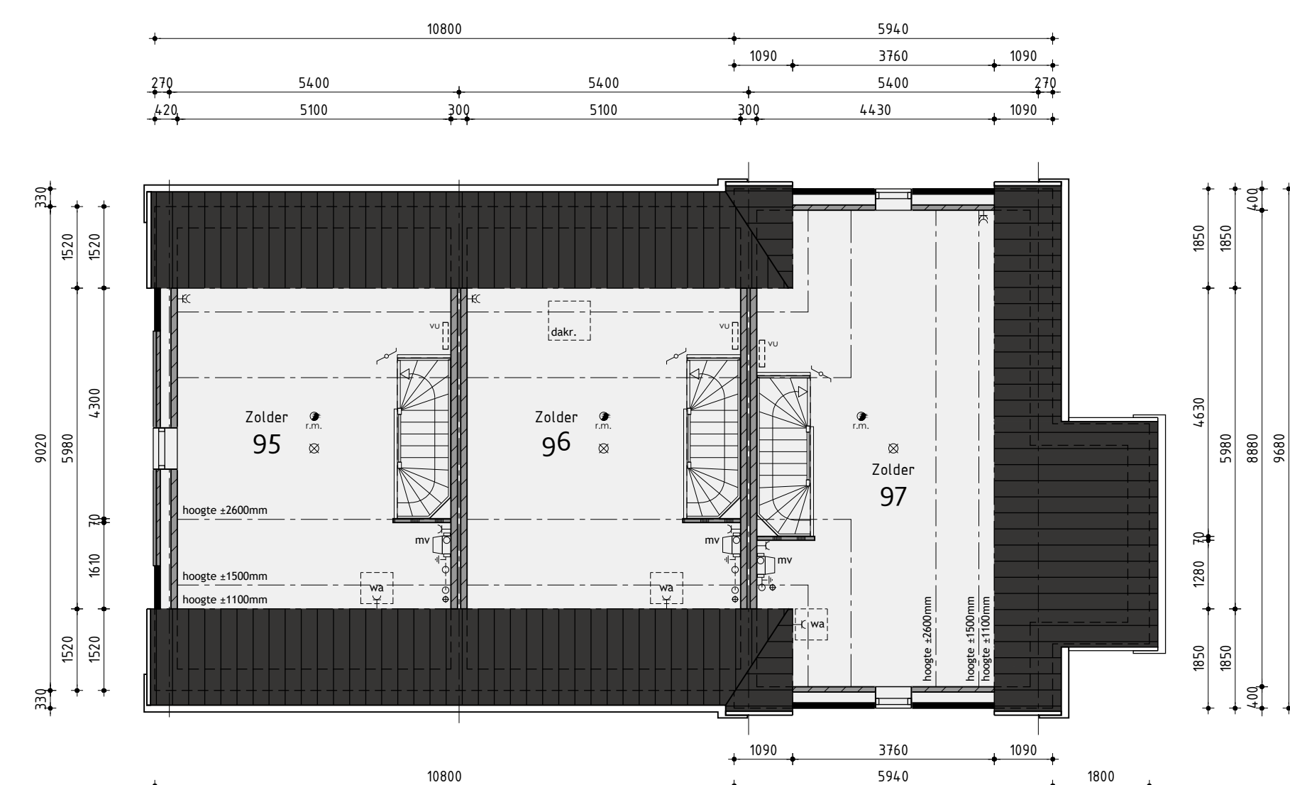
2de Verdieping
