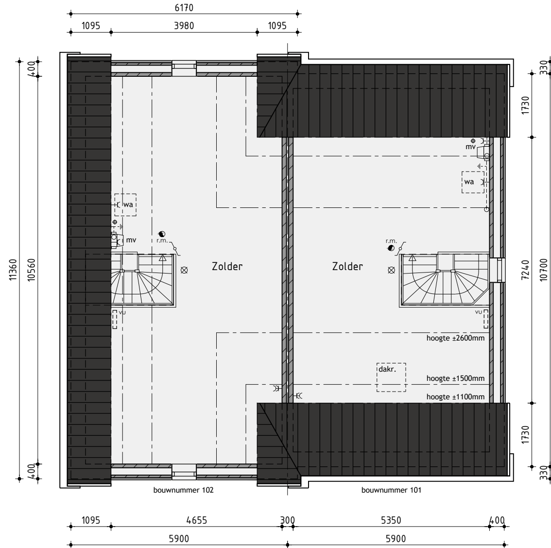
2de Verdieping
