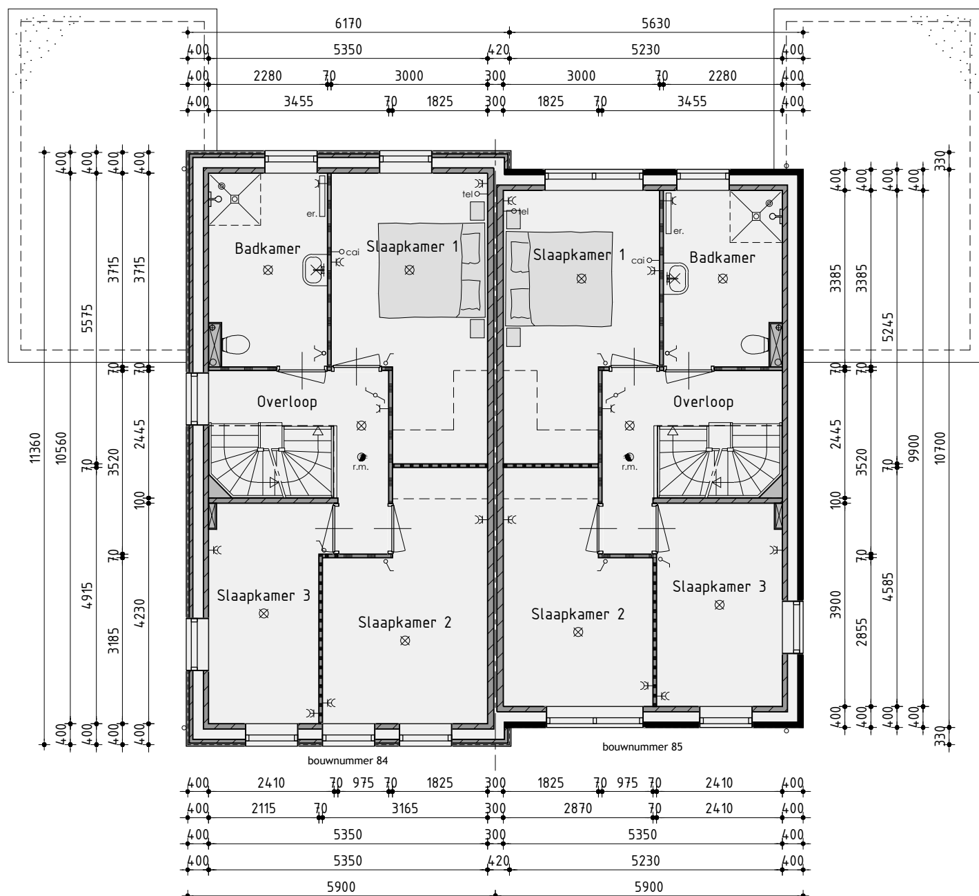
1ste Verdieping
