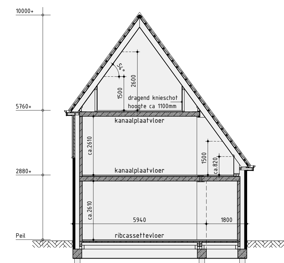
Principe doorsnede B-B
