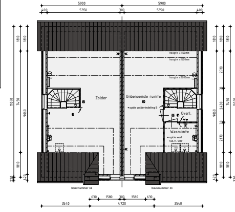
2de Verdieping v.v.z. vloerverwarming
