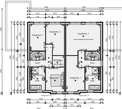
1ste Verdieping v.v.z. vloerverwarming
