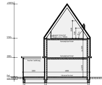
Principe doorsnede A-A
