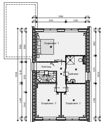
1ste verdieping v.z.v. vloerverwarming
