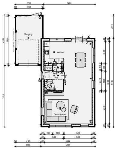
Begane grond v.z.v. vloerverwarming exclusief berging
